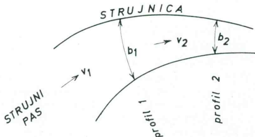
Sl. 9. Strujni pas med sosednjima strujnicama se zožuje proti gradbeni jami
