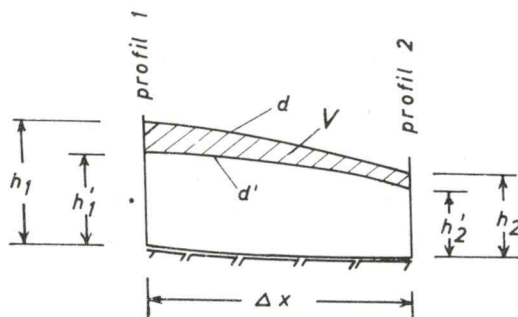
Sl. 11. Skica ponazoruje račun časovnega širjenja depresije
