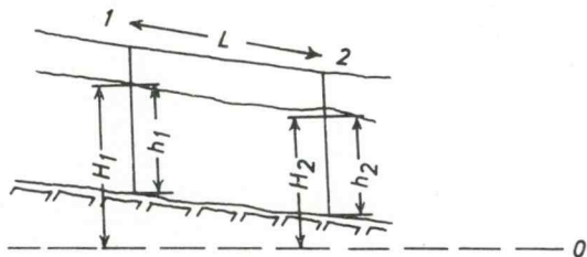
Sl. 10. Tok podtalnice po nagnjeni neprepustni podlagi
