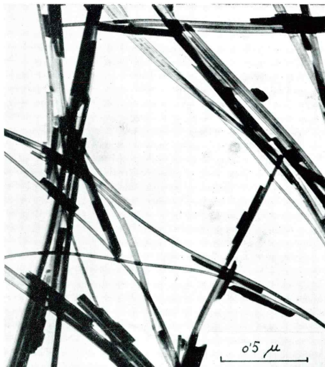
2. sl. Elektronski mikroposnetek stragarskega azbesta pri 45.900-kratni povečavi Fig. 2. Electron microscope picture of the Stragari-asbestos, 45.900 diams.
