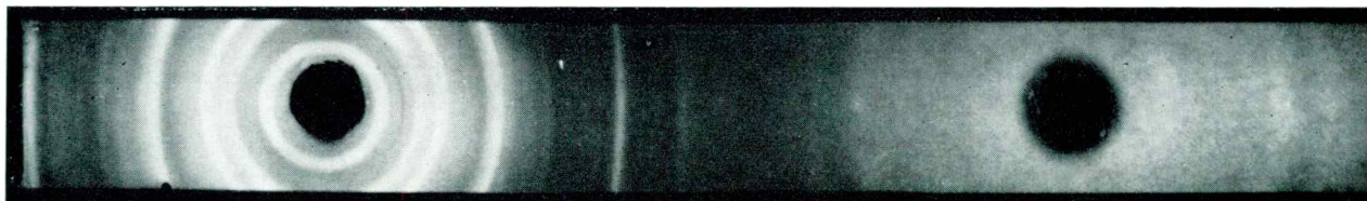
2. sl. Debeygram korlačanskega azbesta z jalovino (kobaltova anoda)
