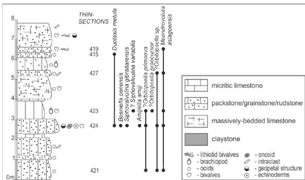
Fig. 4. Grad section with distribution of foraminifera. Sl. 4. Profil Grad z razporeditvijo foraminifer.
