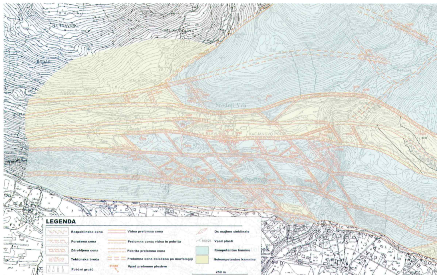
Slika 4. Strukturna karta preiskanega območja.
