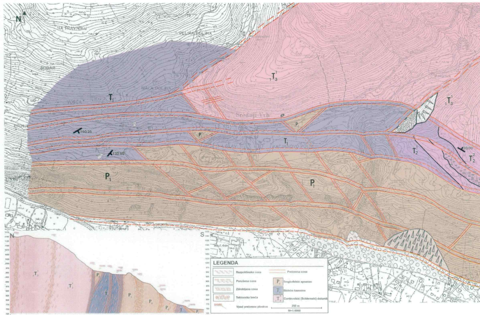
Slika 3. Geološka karta preiskanega območja s tipičnim profilom za raziskano območje. Barve, šrafure in oznake se ujemajo s tistimi na sliki 2. Figure 3. Geologic map and typical depth profile of the investigated area. Colors, patterns and marks correspond to the ones used in Figure 2.
