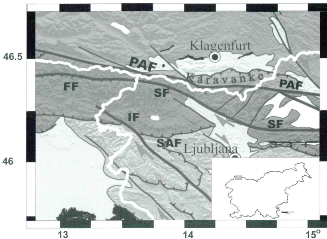
Slika 1. Regionalna strukturna karta območja. SF = Savski prelom; FF = prelom Fella; PAF = Periadriatska prelomna cona; IF = Idrijski prelom; SAF = Južno-alpska nariivna cona. Izsek v desnem spodnjem kotu karte prikazuje preiskano območje s sivim pravokotnikom.
