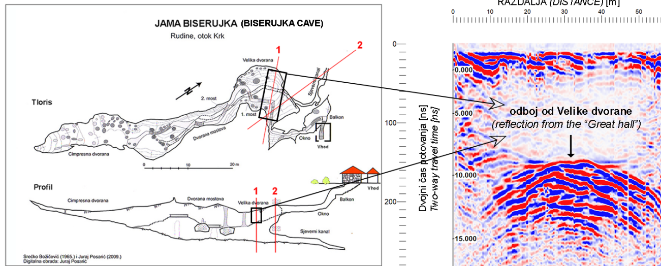
Sl. 9. Primer radargrama nad jamo Biserujko na Krku. Dvorana je velika in polkrožne oblike, zato izmerjeni prečni profil nad jamo povzroči jasno hiperbolično anomalijo.
