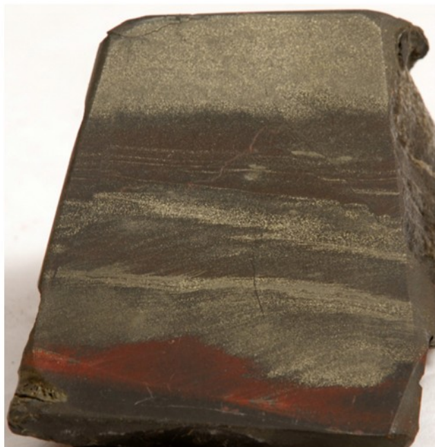
Sl. 9. Sedimentna ruda – opekovka. Navzkrižna laminacija, vzdolžni presek male koritaste plastnatosti. Zgoraj vodoravna laminacija. Kropeč IIm/7. Velikost vzorca 7 x 8 cm. Foto: Jani Peternej
