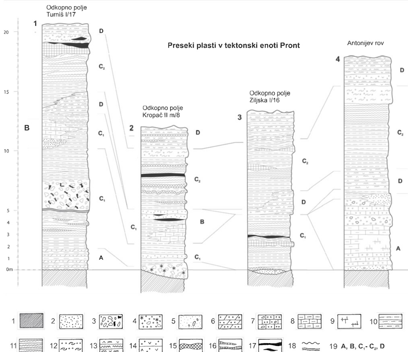
Sl. 3. Profili plasti skoncra v tektonski enoti Pront. 1. karbonski klastiti – skrilavi glinavci, meljeveci in kremenovi peščenjaki; 2. kaolinčne kamnine bogate s piritom; 3. bituminozni dolomitni konglomerat in muljasti konglomerat; 4. dolomitni pečenjak, ponekod prodat; mestoma prepojen s samorodnim živim srebrom (zvezdice) 5. apnenčev dolomitni ali dolomitni apnenčev meljevec, ponekod prodat; 6. bituminozni dolomitni peščenjak in meljevec; 7. peščeni mikritni apnenec, ponekod prodat; 8. laporovec in laporasti apnenec; 9. meljasti mikritni apnenec in mikritni apnenec; 10. bituminozni dolomitni ( C_1 ) ali kremenov ( C_2 ) peščenjak; 11. skrilavi bituminozni dolomitni ( C_1 ) ali kremenov ( C_2 ) meljevec, skrilavi glinavec z vložki radiolarijskega roženca; 12. glinenčevo-litični kremenov peščenjak z ostanki lupin brachiopoda Discina ; 13. piroklastiti z roženca; 14. tufski peščenjak; 15. plasti in leče pirita; 16. bogato orudenje – jeklenka; 17. leče premoga (antracita); 18. erozijska in drsna površina; 19. litološka zaporedja
