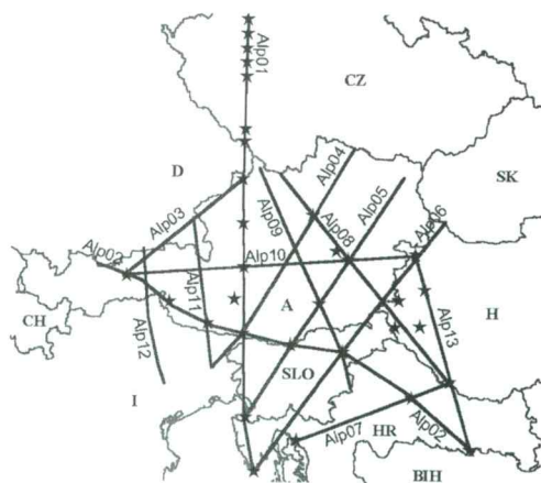
Sl. 2. Položaj seizmičnih profilov in strelnih točk projekta Alp 2002
