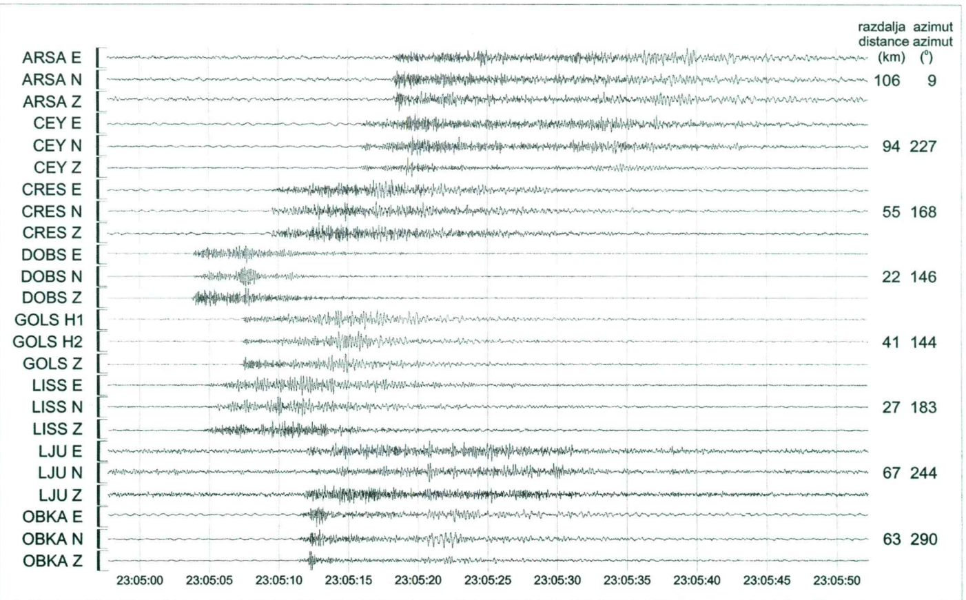
Sl. 6. Zapis eksplozije na strelni točki pri Vojniku na šestih potresnih opazovalnicah v Sloveniji in dveh v Avstriji. Lokacije opazovalnic so na sliki 3 Fig. 6. Record of explosion at the shot point Vojnik on six seismological stations in Slovenia and two in Austria. Locations of seismological stations are shown in Fig. 3
