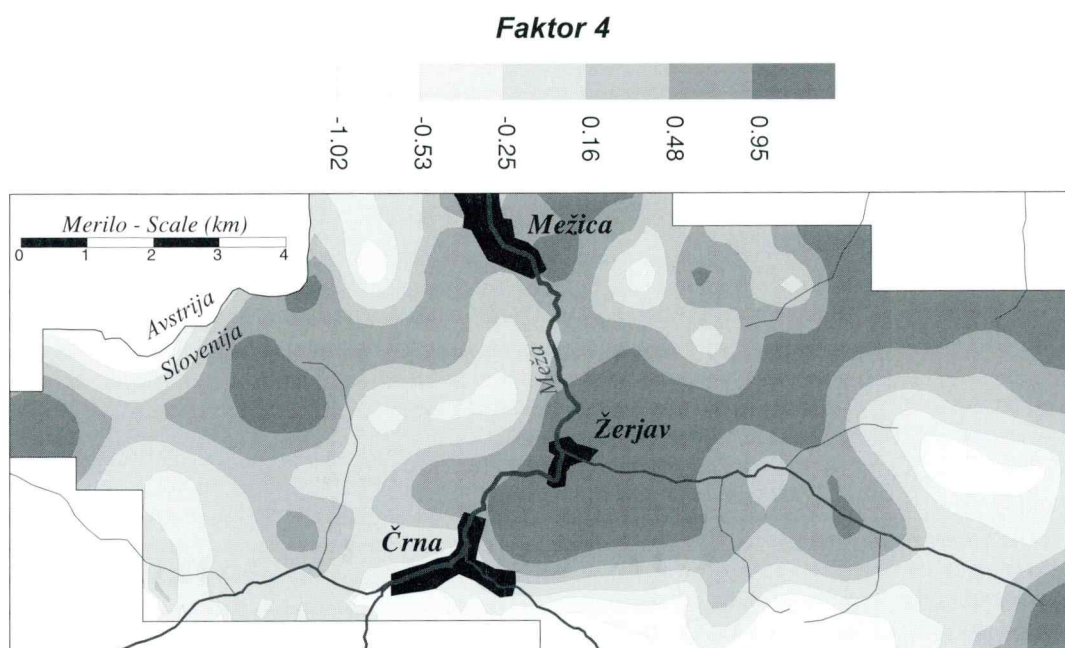
Sl. 4b. Porazdelitev faktorja 4 (Pb in Zn) v spodnjih talnih horizontih
