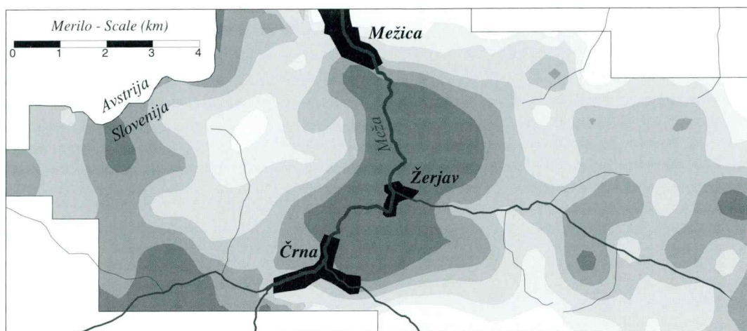
Sl. 4a. Porazdelitev faktorja 4 (Pb in Zn) v vrhnjem talnem horizontu
