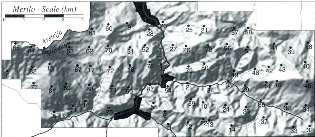
Sl. 2. Digitalni model reliefa območja Mežice z lokacijami vzorčenja v talnih profilih Fig. 2. Digital relief model of Mežica area with soil profile locations
