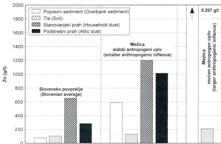
Sl. 6. Porazdelitev vsebnosti Zn v vzorčnih sredstvih na območju Mežice
