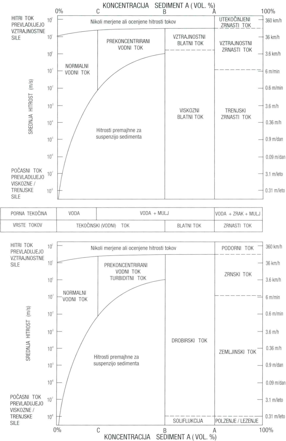
Sl. 3. Reološka klasifikacija tokov zmesi sediment - voda/zrak in ustrezna uporaba obstoječe terminologije tokov. Za razlago glej tekst (prirejeno po Pierson & Costa, 1987).
