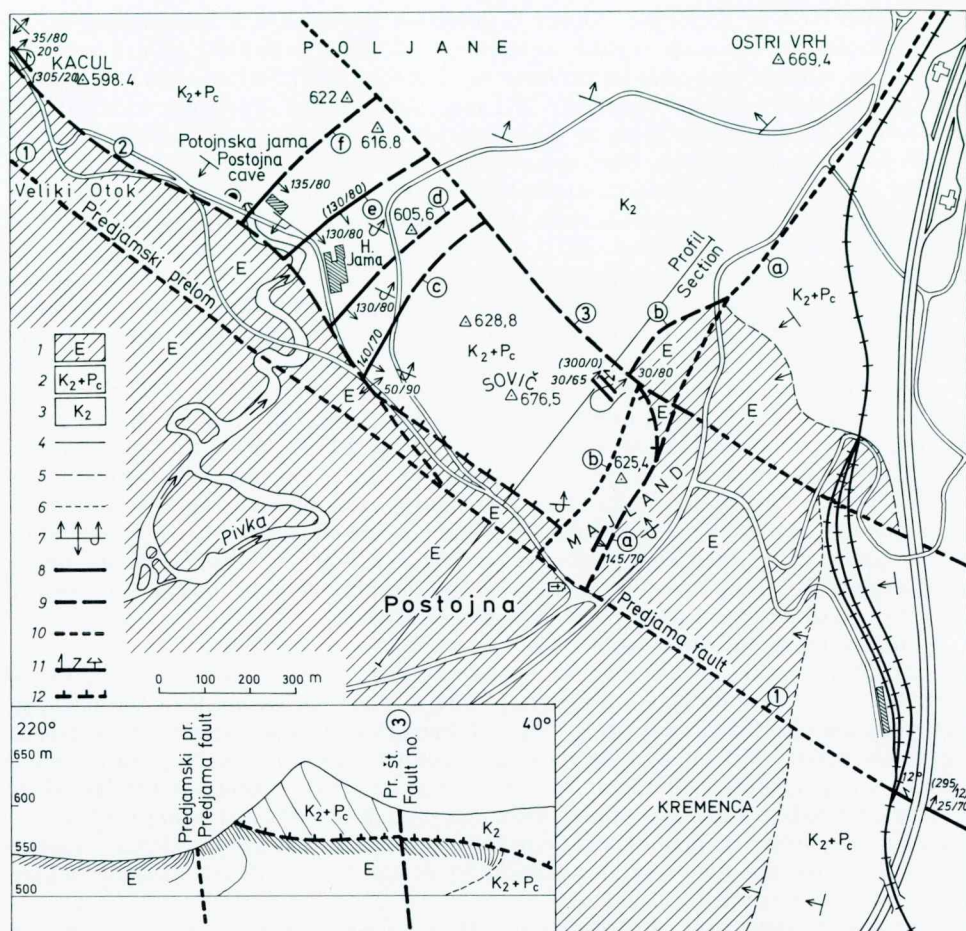
Sl. 1. Skica geološke zgradbe Postojne in bližnje okolice
