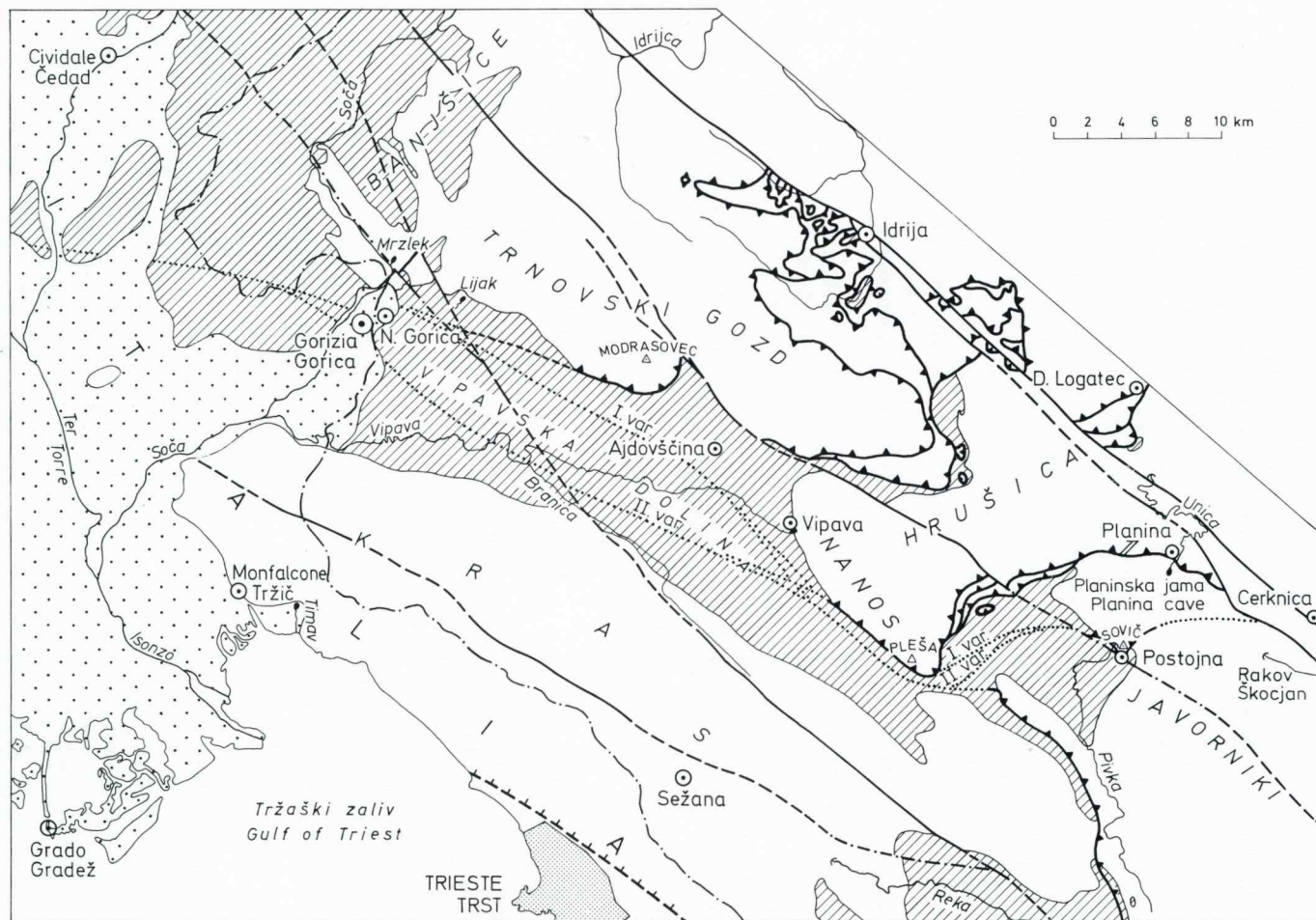
Sl. 4. Tektonska zgradba Komenske planote (Kras) in Visokega krasa (Banjšice, Trnovski gozd, Nanos, Hrušica) jugozahodno od Idrijskega preloma. Legenda na sl. 2 in 3
