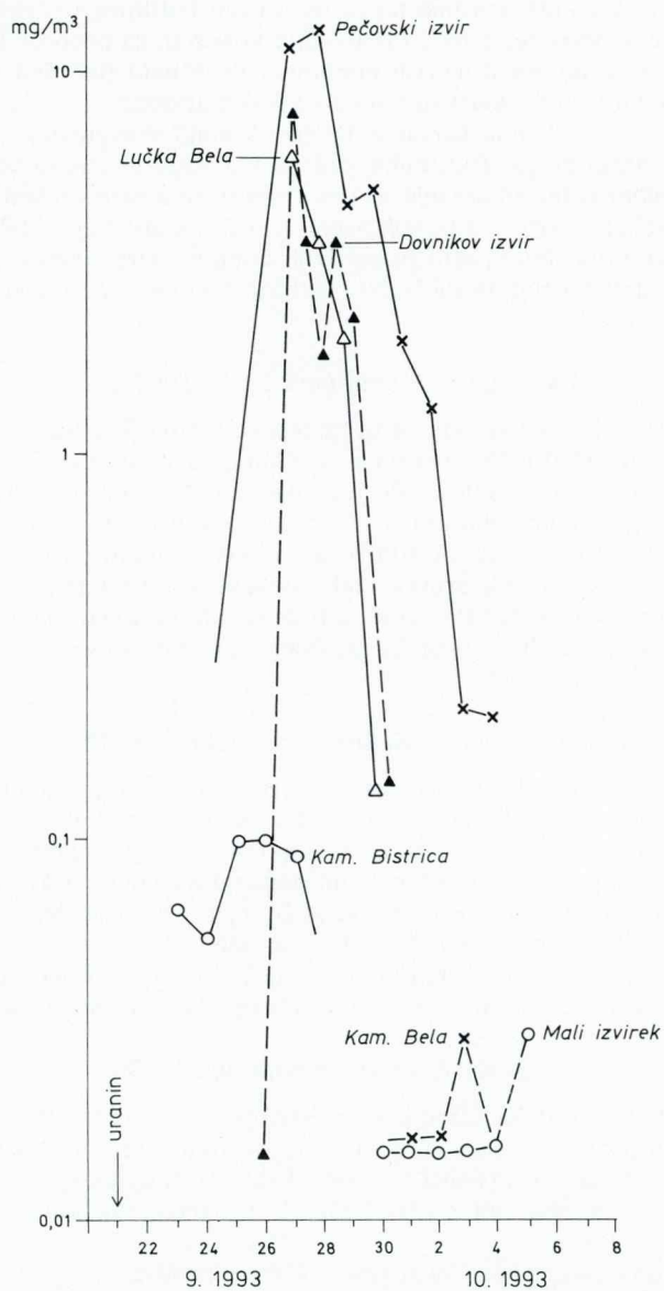
Sl. 4. Krivulja koncentracij uranina pri barvanju na Korošici
