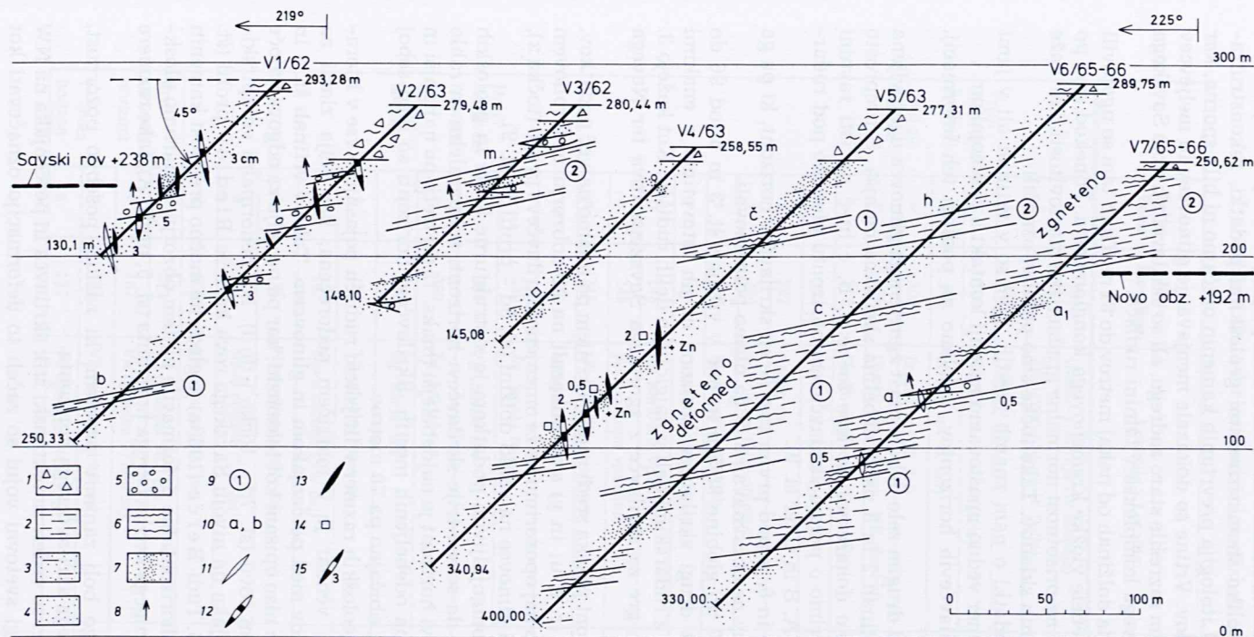
Sl. 6. Rudišče Litija, rezultati raziskovalnega vrtanja (prirejeno po podatkih Fabjančiča, 1964)
