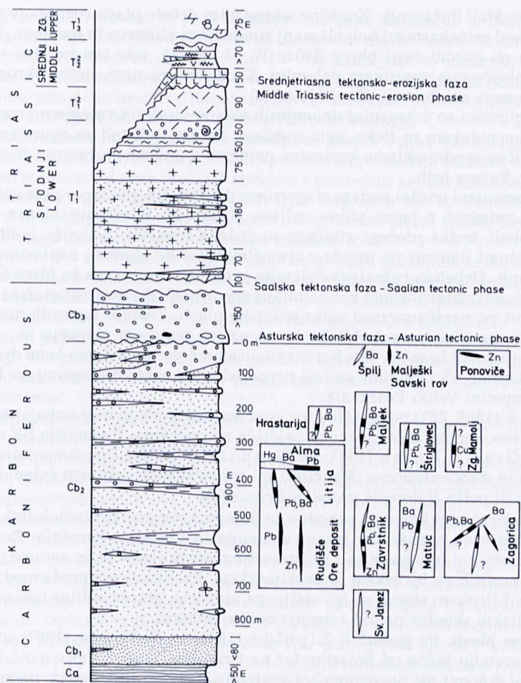
Sl.3. Geološki stolpec območij Litija-Šmartno in Maljek
