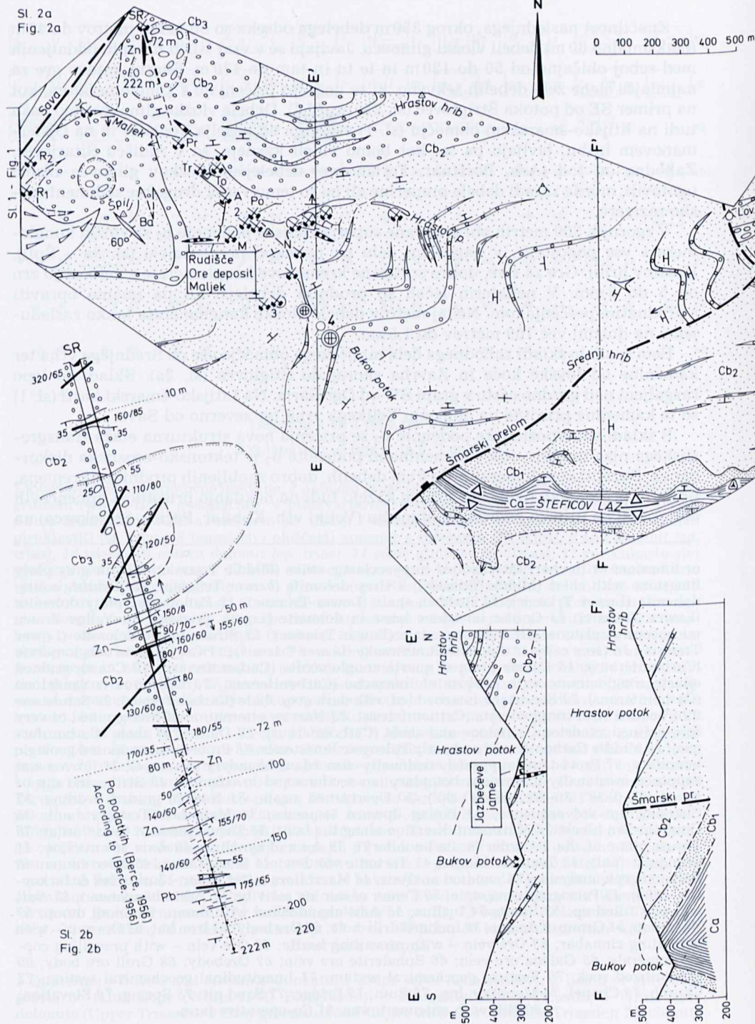
Sl. 2a. Geološka karta in prerezi območja Maljek Sl. 2b. Geološke razmere v Savskem rovu (SR)
