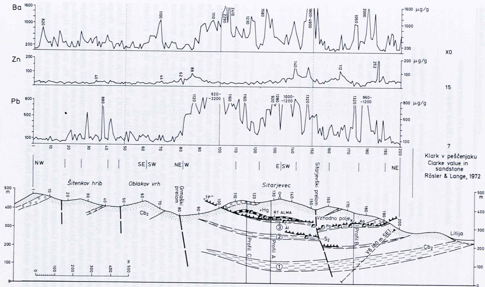
Sl. 9. Geokemični profil vzdolž grebena Sitarjevec-Šitenkov hrib Fig. 9. Geochemical section along Sitarjevec-Šitenkov hrib hillock
