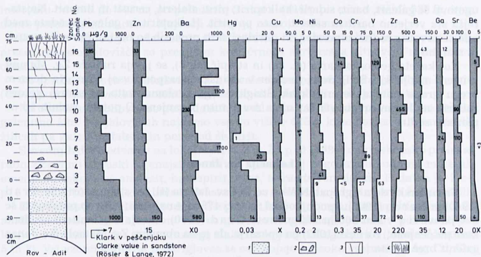
Sl. 8. Porazdelitev prvin po vertikali na profilu SI 1 kremenov pesčenjak; 2 preperina s košči pesčenjaka; 3 preperina s koreninicami; 4 travnata ruša
