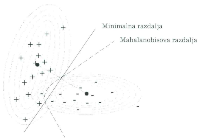
Sl. 5. Različne metode različno delijo podatkovni prostor
