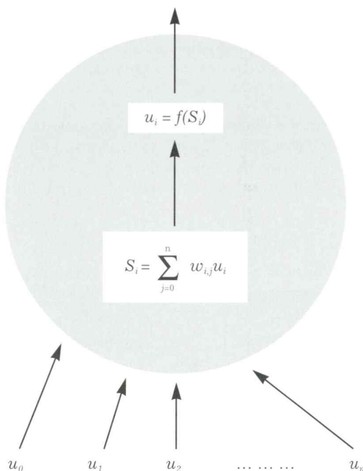
Sl. 10. Umetni nevron - preklopna celica (Gallant, 1993)
