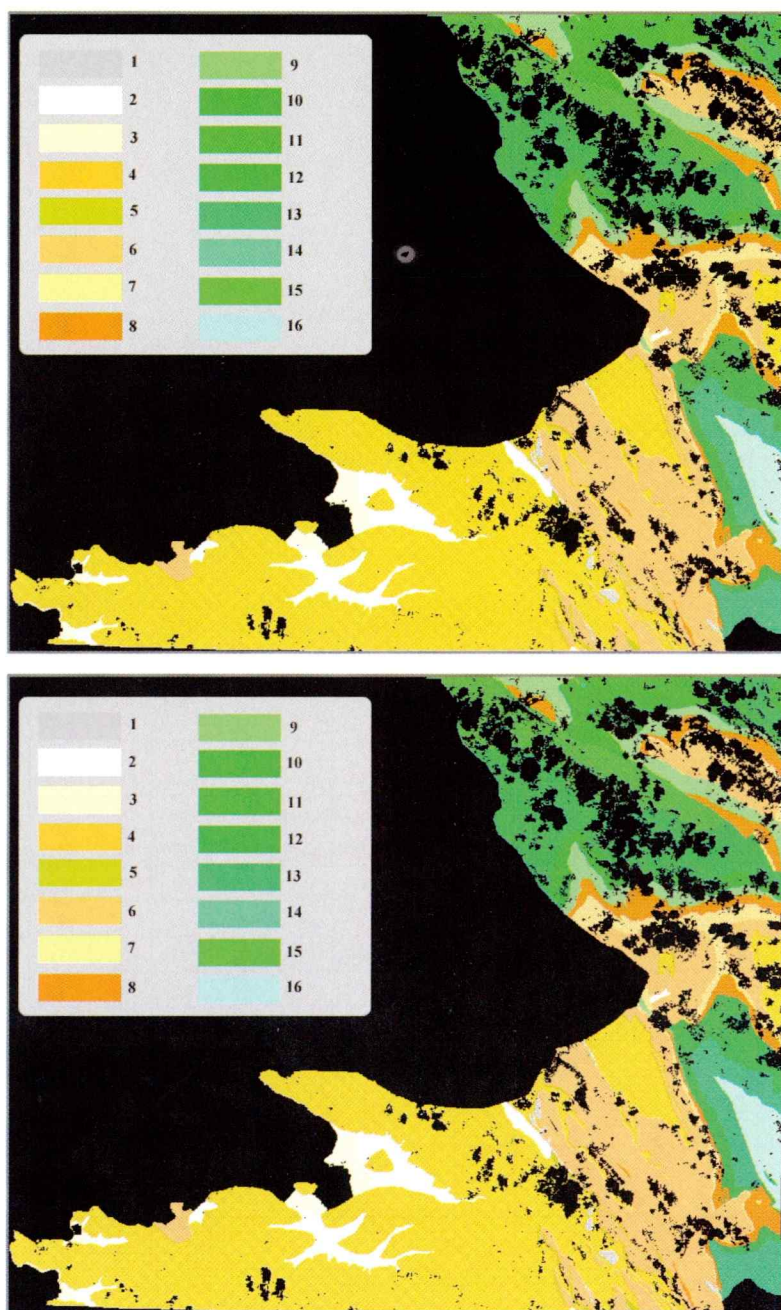
Sl. 6. Geološka karta Slovenskega Primorja (zgoraj) in rezultat nadzorovane klasifikacije po metodi največje podobnosti za 16 razredov (spodaj)
