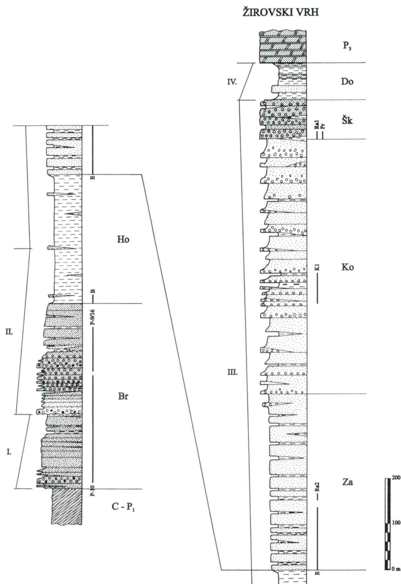
Sl. 2. Litostratigrafski razvoj Grödenske formacije na območju Žirovskega vrha z lego vzorčevanih profilov P-10, Pr-9/16, Kl, Ra1, projiciranih profilov B, E z območja Sovodnji, Ra2 z območja Golega vrha in Pr z območja Smrečja. Na levi strani so prikazani izdvojeni makrocikli. Osenčeni del profila označuje sivo in zeleno obarvane kamnine
