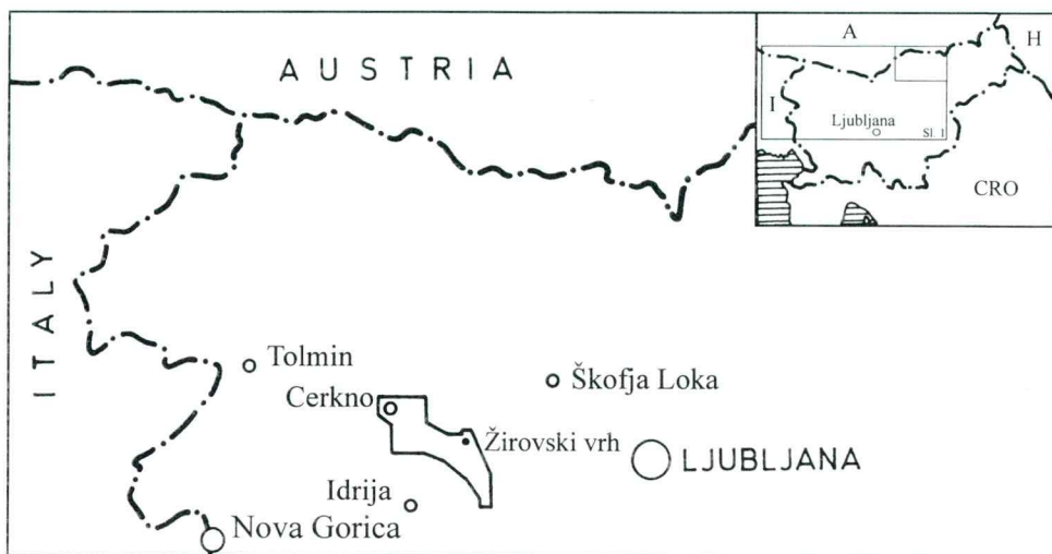
Sl. 1. Situacijska karta širšega raziskovalnega območja, ki ga je podrobno geološko skartiral Mlakar (1979 - 1982)
