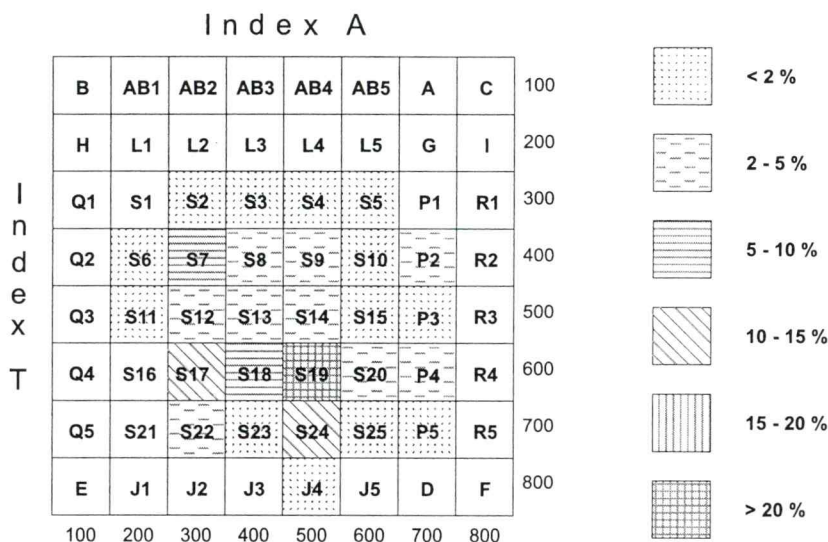
Sl. 10. Tipološka frekvenčna porazdelitev cirkona v grödenskem peščenjaku
