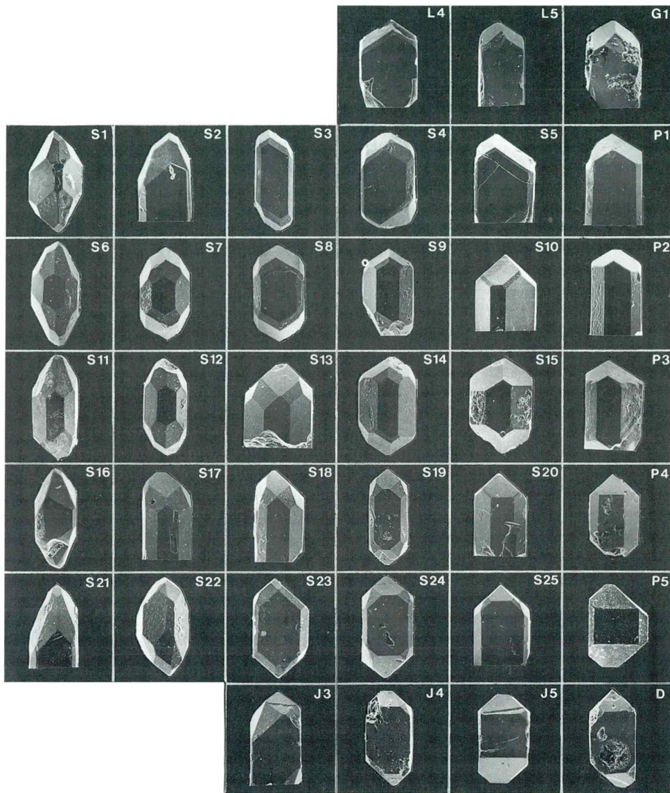
Sl. 4. Tipološke oblike cirkona ugotovljene v grödenskem peščenjaku Fig. 4. Typologic forms of zircon found in the Val Gardena sandstone
