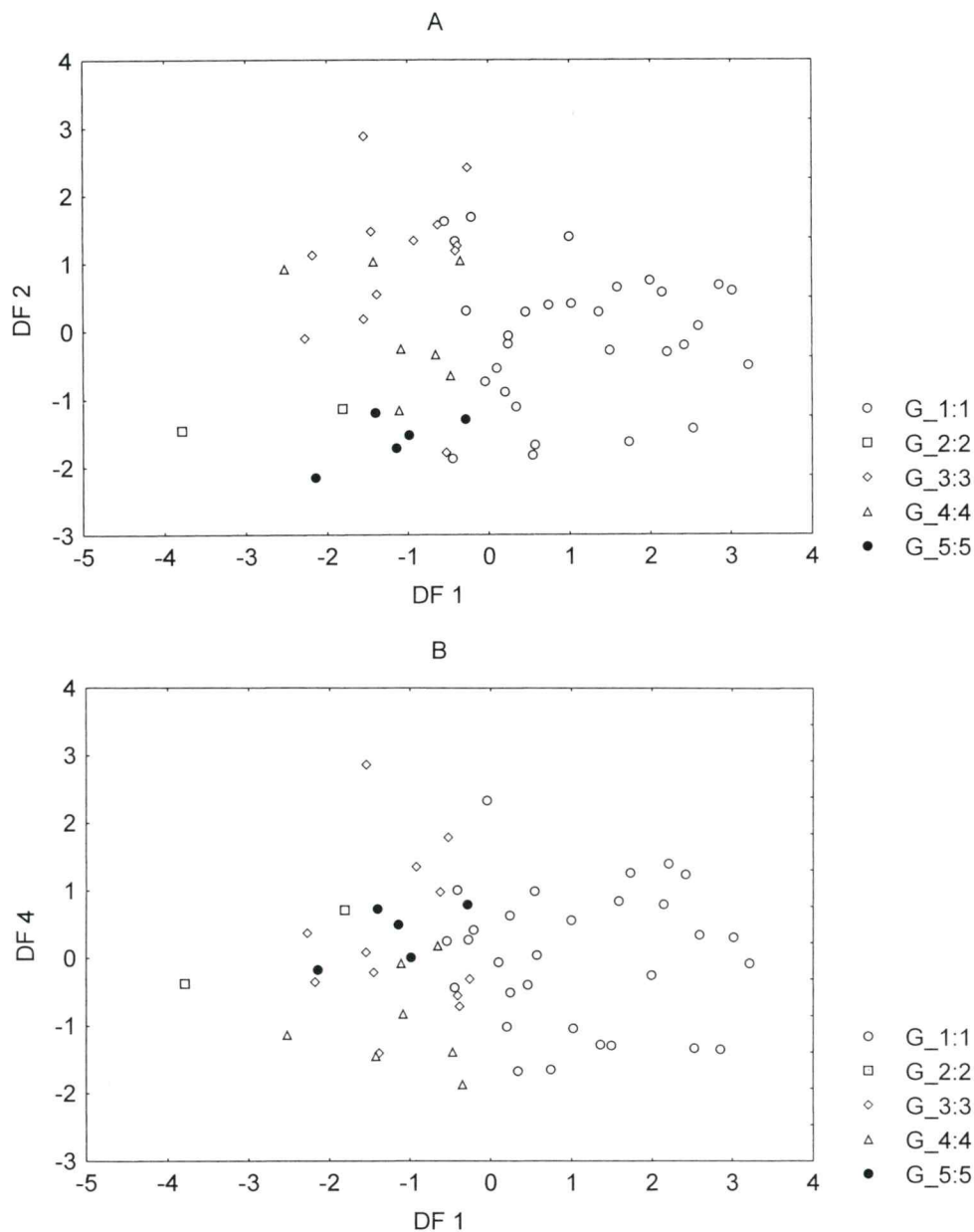
Sl. 8. Bivariatna diagrama standardiziranih diskriminatnih funkcij A. DF1 - DF2 in B. DF1 - DF4, ki ločujejo enote (vzorke) litostratigrafskih členov (1 - Brebovniški člen, 2 - Hobovski člen, 3 - Zalski člen, 4 - Koprivniški člen, 5 - Škofješki člen)
