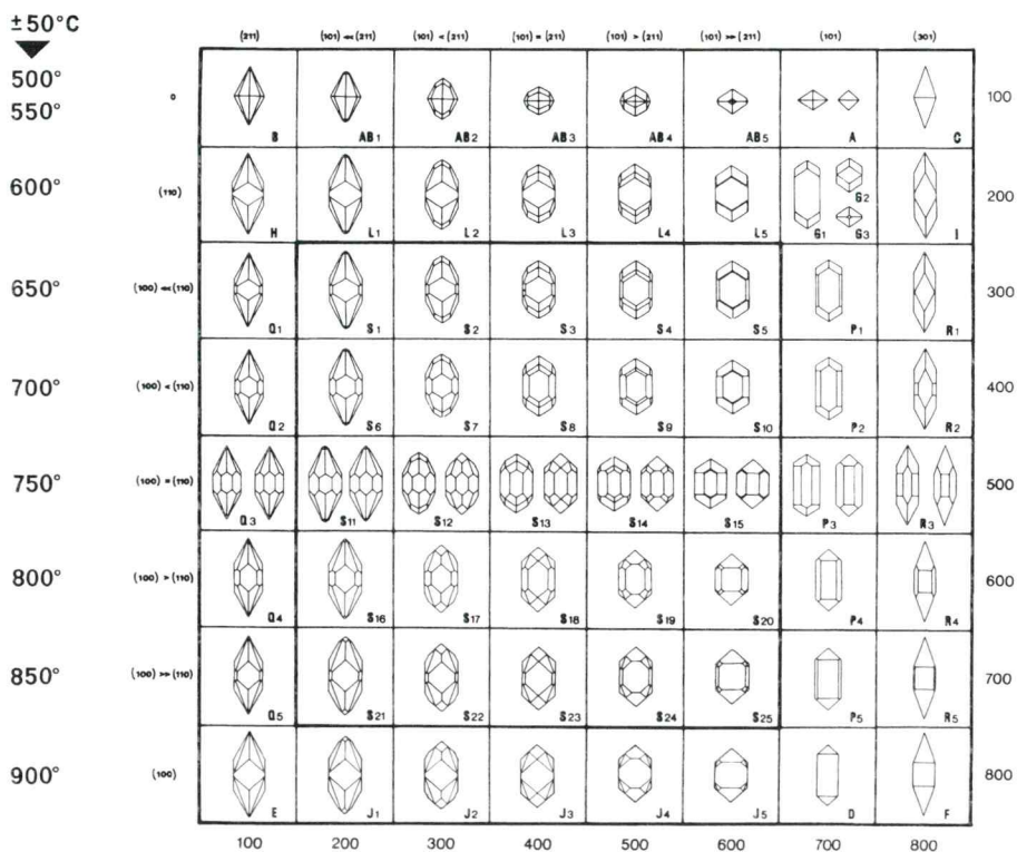
Sl. 3. Pupinova tipološka klasifikacija cirkonov (prirejeno po P u p i n-u, 1980, 20, Fig. 1)
