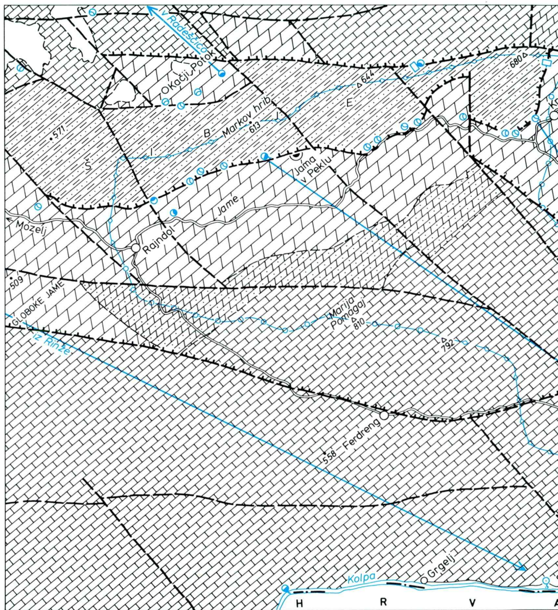
Sl. 1. Geološka karta območja Šumetca (Savić & Dozet, 1985)
