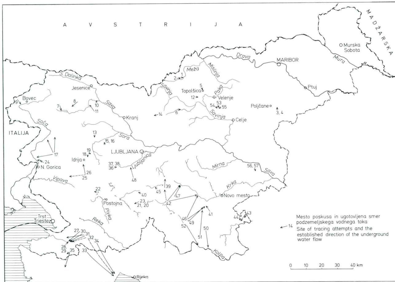
Sl. 1. Smeri tokov kraških podzemeljskih voda v Sloveniji Fig. 1. Directions of karstic underground waters in Slovenia
