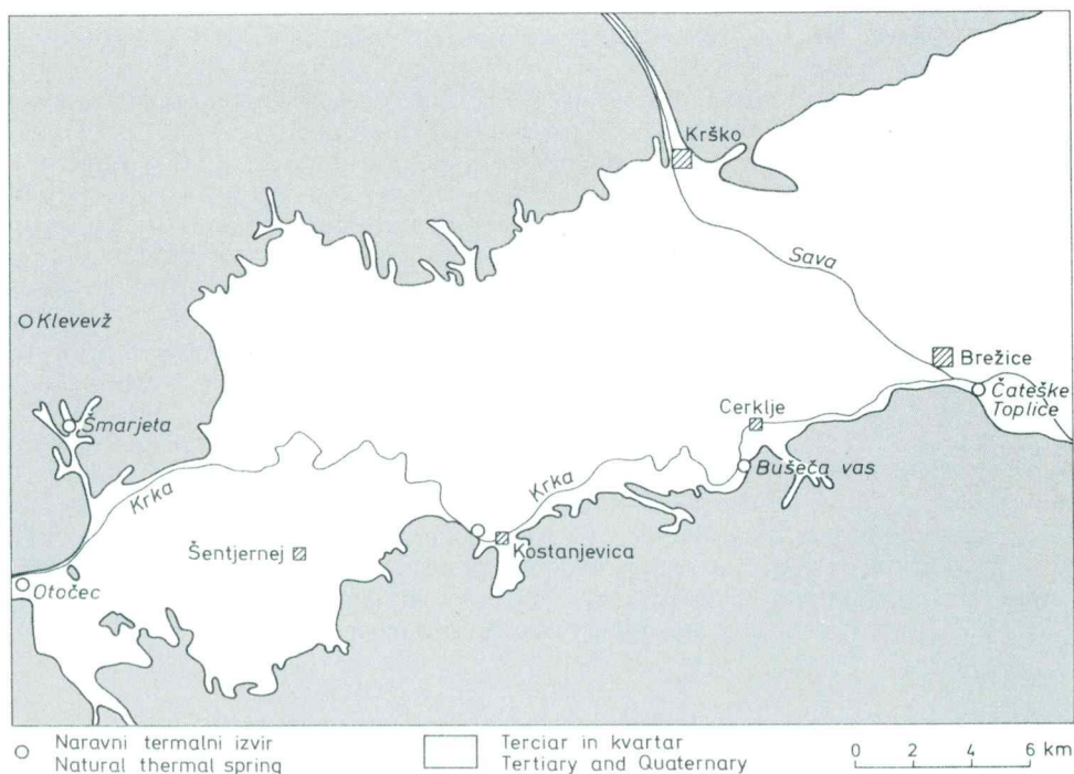
Sl. 1. Karta termalnih izvirov v Krško-Brežiški kotlini
