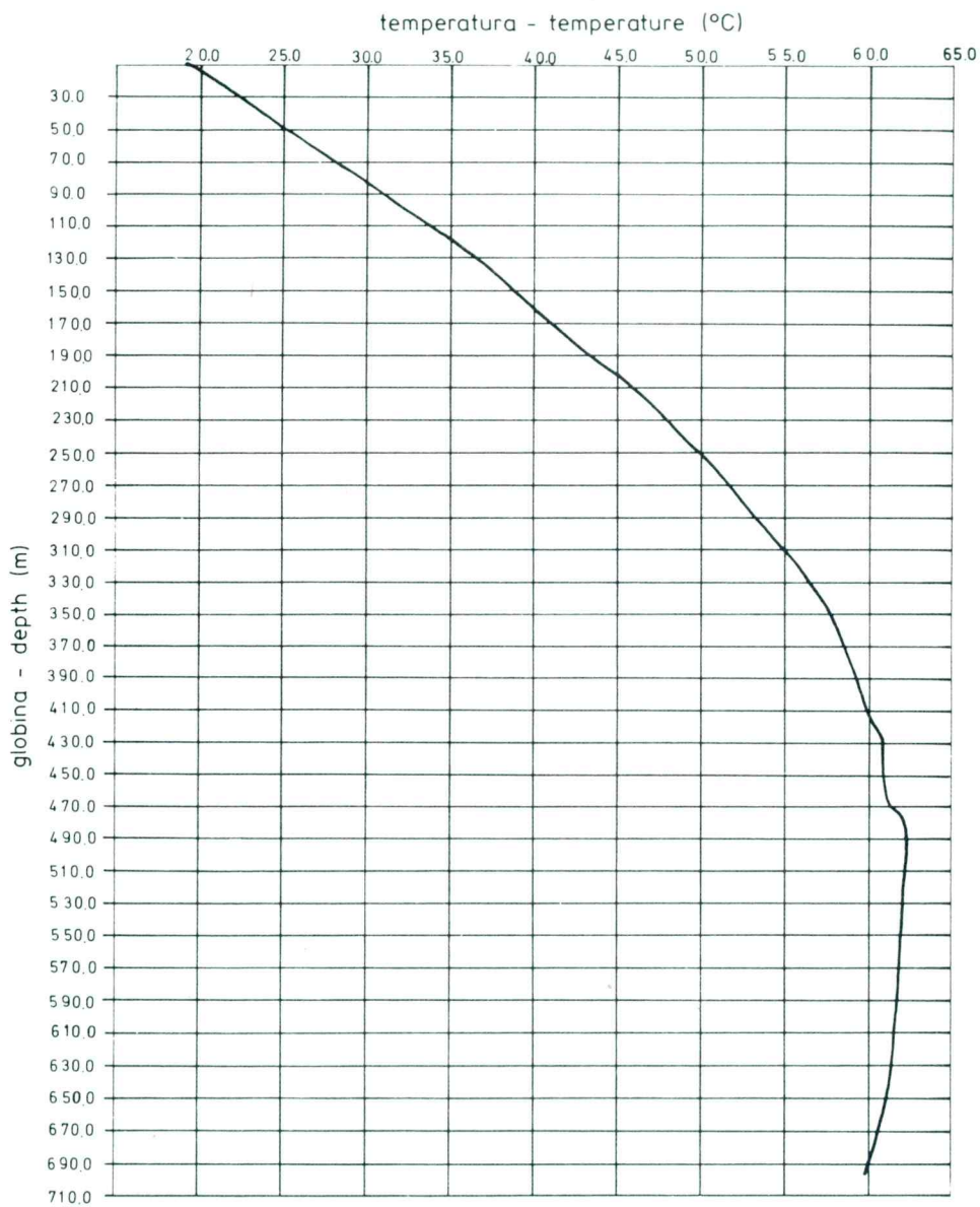
Sl. 2. Termogram vrtine L-1/86 pri Mostecu
