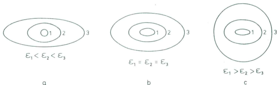
Fig. 1. Three macroseismic field models Sl. 1. Trije modeli makroseizmičnega polja
