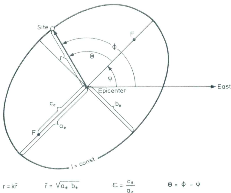
Fig. 2. The parameters of an elliptic macroseismic field Sl. 2. Količine eliptičnega makroseizmičnega polja
