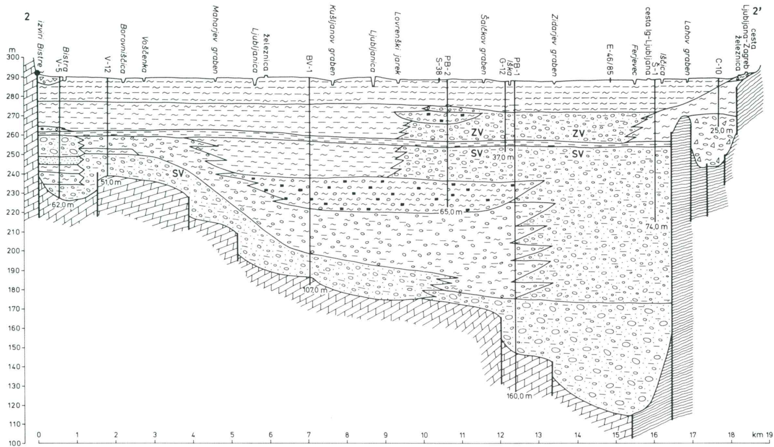
Sl. 5. Vzdolžni profil 2-2' čez južni del Ljubljanskega barja
