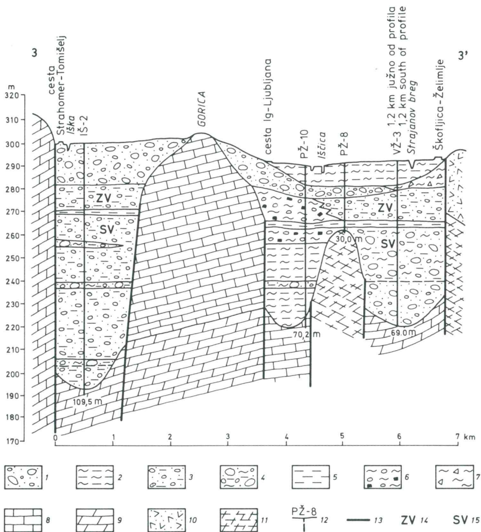
Sl. 6. Prečni profil 3-3' čez vršaja Iške in Želimeljščice
