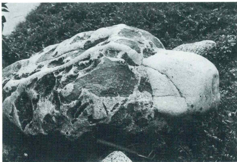
Sl. 2. Intruzivna magmatska breča. Drobnozrnati mafični magmatski vključki v porfiroidnem granitu. Oboje seče mlajša drobnazrnata granitna žila
