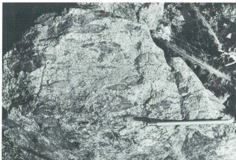
Sl. 5. Raztrgani drobci kontaktno metamorfnega skrilavca v granitoidni kamenini, ki tudi predstavlja intruzivno brečo
