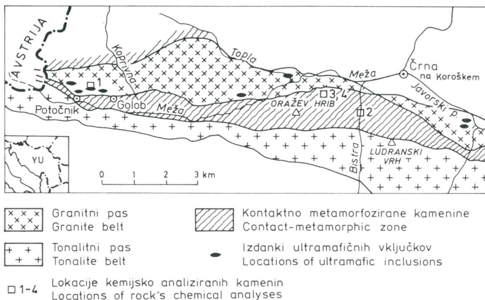
Sl. 1. Del karavanške magmatske cone zahodno od Črne na Koroškem (prirejeno po Tellerju, 1898)
