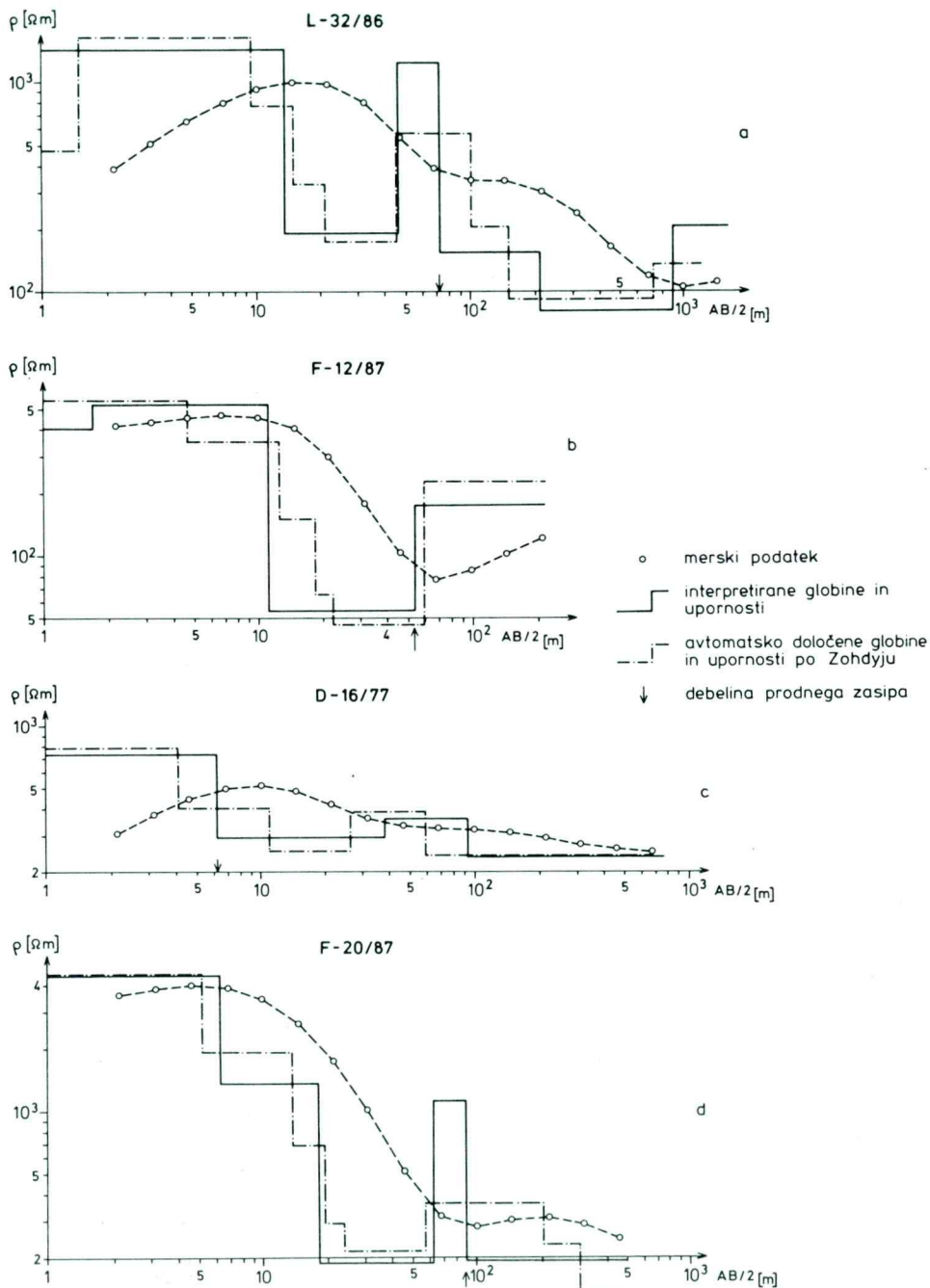
Sl. 2. Primeri geoelektričnih sond z interpretacijo
