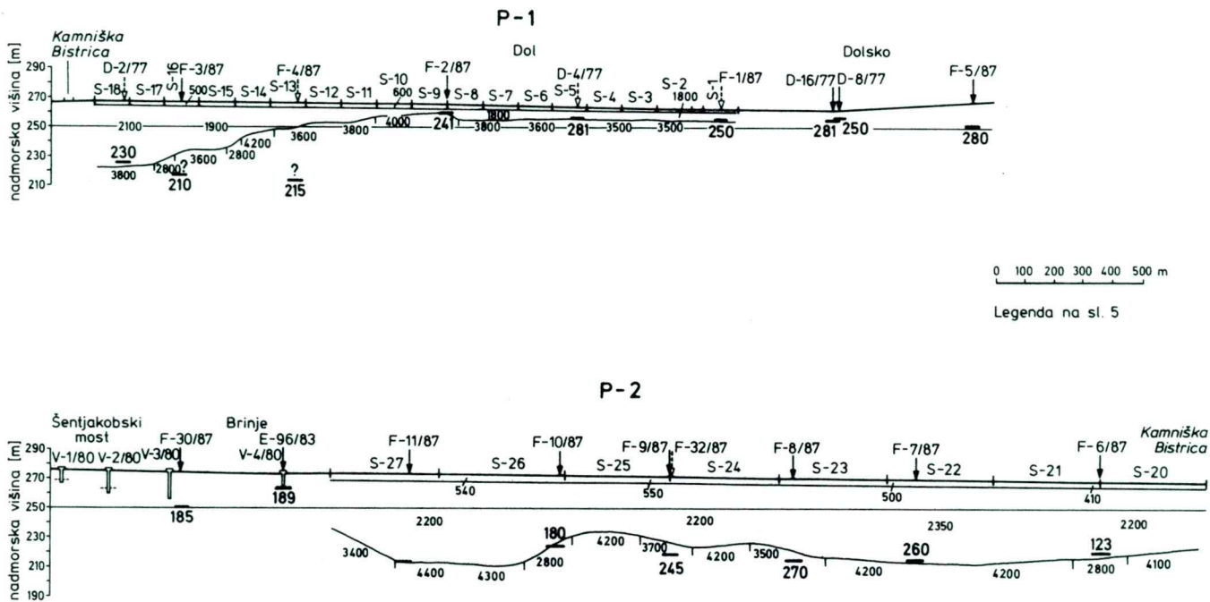
Sl. 3. Geofizikalna profila P-1 in P-2
