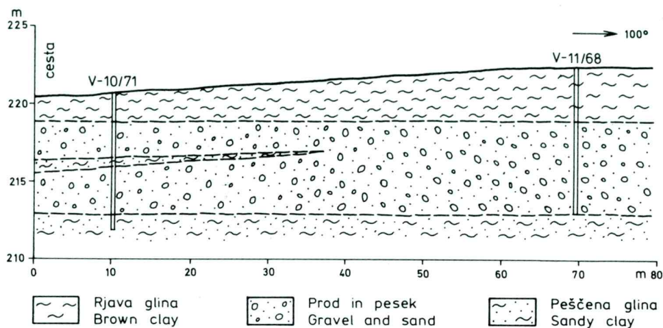
Sl. 2. Geološki profil dela nahajališča kremenovega prod in peska v Puconcih
