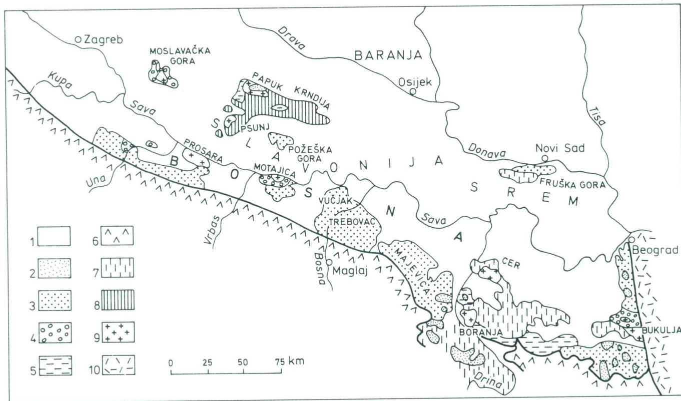
Sl. 1. Pregledna geološka karta dodirnog područja sjevernih Dinarida i Panonskog strukturnog kompleksa
