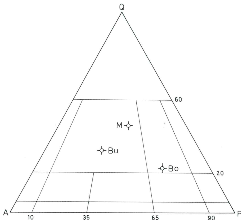
Sl. 2. Srednji modalni sastavi granitoidnih stijena Motajice-M, Bukulje-Bu i Boranje-Bo
