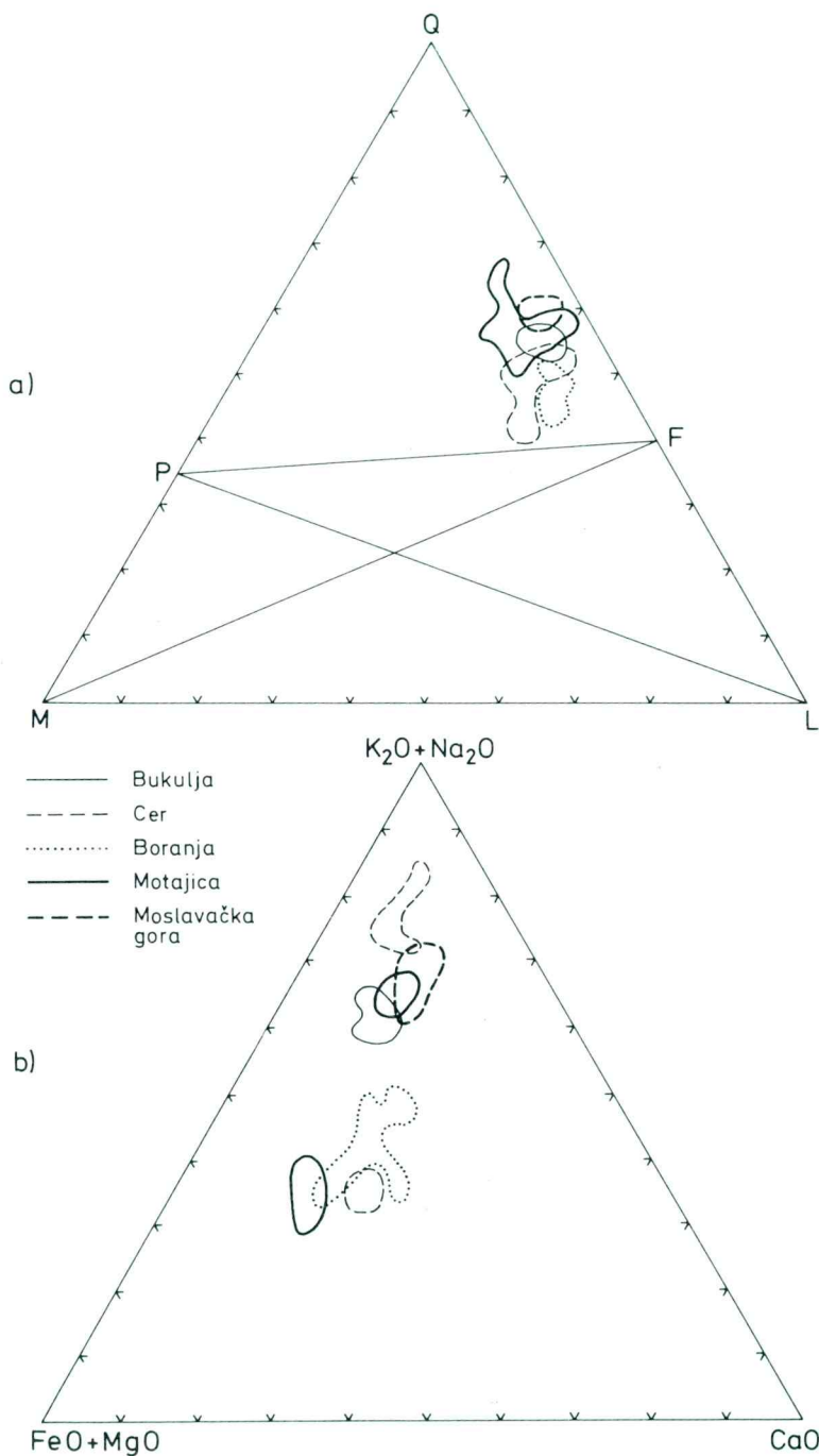
Sl. 3. QLM (a) i K_2O+Na_2O - FeO+MgO - CaO (b) trokomponentni dijagrami za stijene granitne asocijacije
