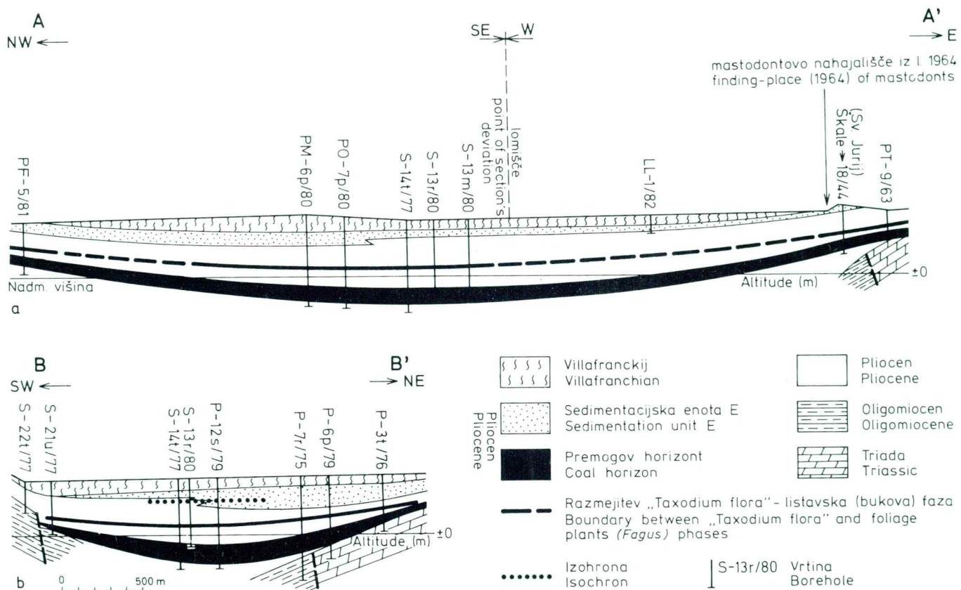
Sl. 14. Geološka prereza
