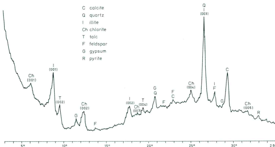
Sl. 12. Rentgenogram orientiranega preparata glinaste frakcije recentnega sedimenta; vzorec jedra iz vrtine V-6/79
