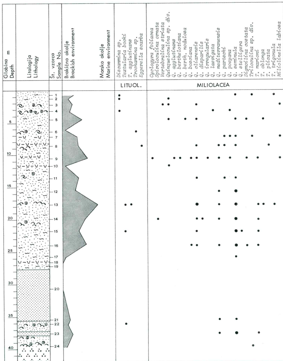
Sl. 13. Združba foraminifer, določena v vzorcih jedra vrtine V-6/79
