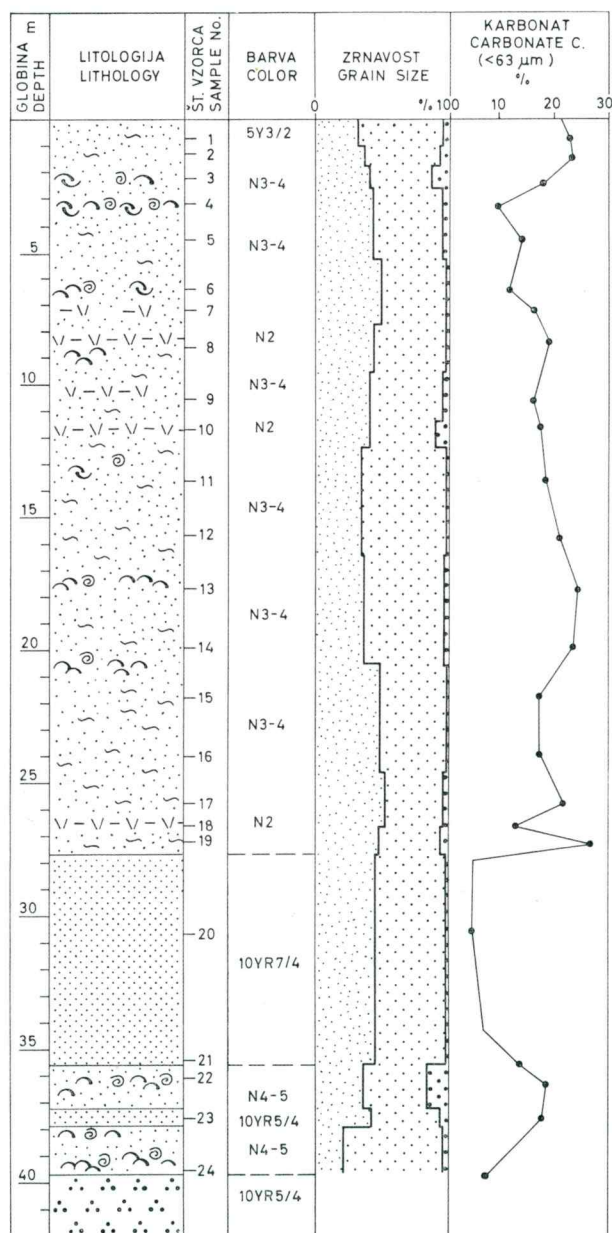
Sl. 9. Litologija, zrnavaost in vsebnost karbonata v vzorcih jedra iz vrtnice V-6/79, soline Lera
