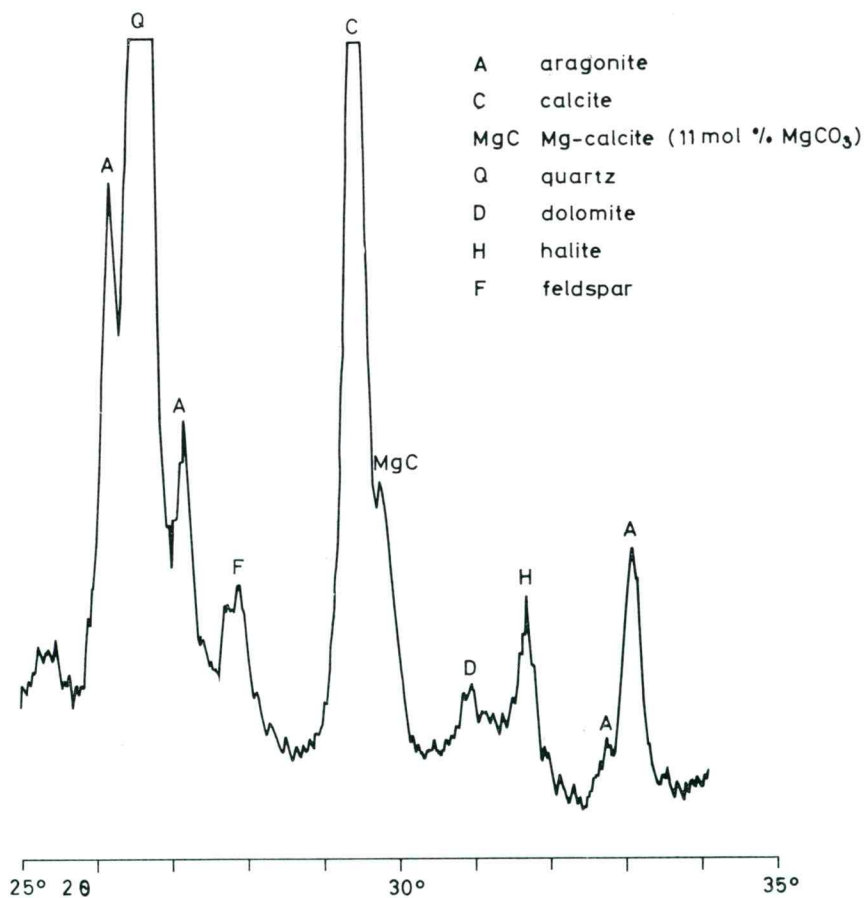
Sl. 5. Rentgenogram vzorca algine skorje, lokacija št. 2, soline Lera
