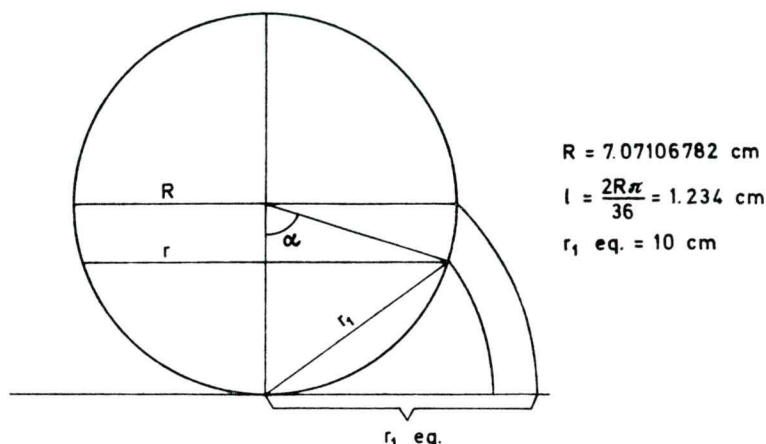
Sl. 1. Parametri osnovne polkrogle
