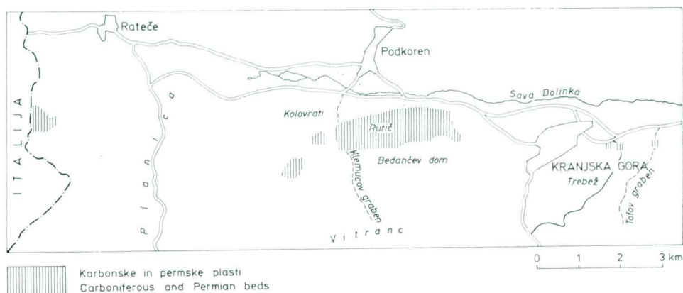
Sl. 1. Razširjenost karbonskih in permskih plasti v severnih Julijskih Alpah Fig. 1. Distribution of Carboniferous and Permian beds in the northern Julian Alps
