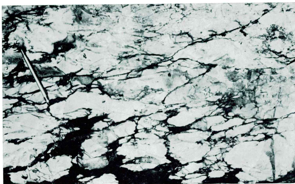
Sl. 5. Žilice sadre (sivo) v anhidritu (belo) na obrobju sulfatne leče. Rudišče Ljubevč Fig. 5. Gypsum veinlets (gray) crossing anhydrite (white) on the margine of the sulphate lens. Ljubevč mine
