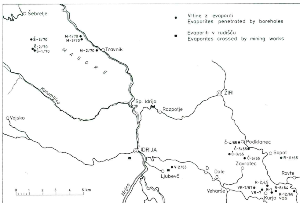
Sl. 1. Skica ozemlja s pojavi evaporitov na Idrijskem Fig. 1. Location map showing the evaporite occurrences in the Idrija region
