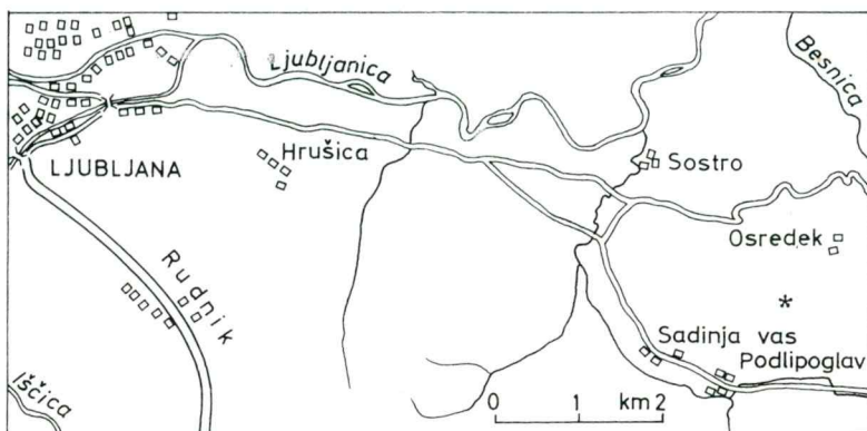
Sl. 1. Položaj trogkofelskega konglomerata pri Podlipoglavu* Fig. 1. Location map of Trogkofel-Conglomerate at Podlipoglav*
