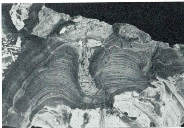
Sl. 10. Stromatolitni horizont prerašča intraformacijsko brečo. Posamezni intraklasti so inkrustirani z algami. Reto-lias, Grmače, naravna velikost
