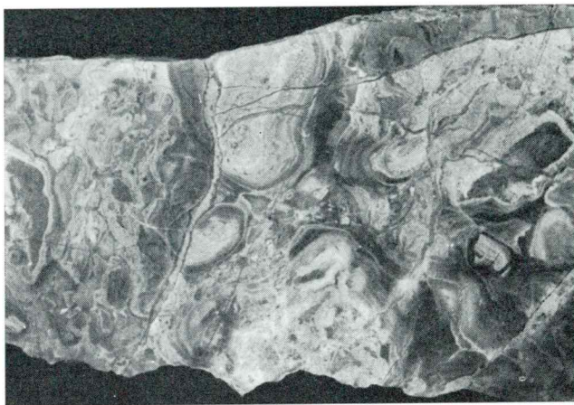
Sl. 12. Intraklasti mikritnega apnenca so inkrustirani z algami. Reto-lias, Grmače, naravna velikost
