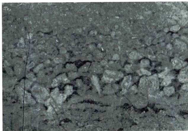
Sl. 4. Intraklasti, inkrustirani z algami v mikritnem dolomitiziranem apnencu s peleti. Anizično-ladinski dolomit, kamnolom Lukovica, naravna velikost
