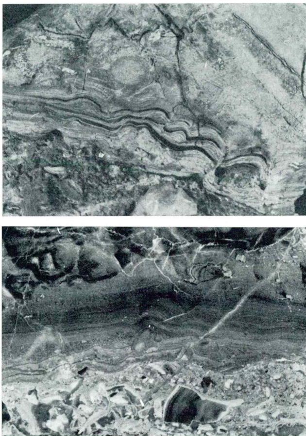
Sl. 11. Intraformacijska breča prehaja v stromatolit in mikritni apnenec. Spodaj: presek, zgoraj: naravna površina. Reto-lias, Grmače, naravna velikost
