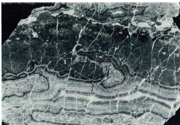
Sl. 8. Korozijske votline v mikritnem apnencu, zapolnjene s pasovitim sparitom, kažejo kokardno teksturo. Zgornjetriadni apnenec, Črni graben, \frac{1}{2} naravne velikosti
