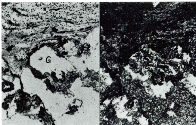
Sl. 9 levo. Siderit obroblja v kaolinit spremenjen glinenec (G). Spodaj kaolinitno pšeno, zgoraj vezivo. 80 m SE od slepega jaška Center, II. medobzorje. Presevna polarizirana svetloba, povečava 30 \times . 9 desno. Isto, le pri navzkrižnih nikolih
