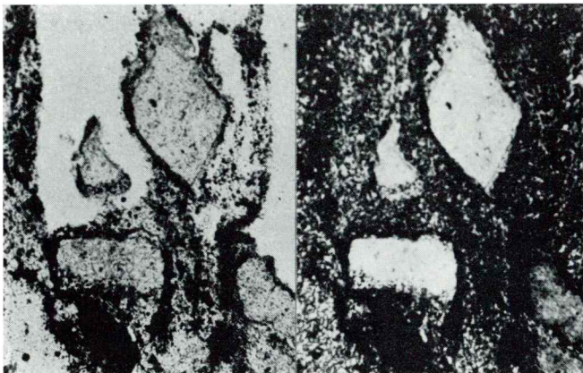
Sl. 10 levo. Drobna pirithna zrna obrobljajo siderit, leže pa tudi v kaolinitnem pšenu in v vezivu. Pri slepem jašku št. 16, II. obzorje, vzorec 5. Presevna polarizirana svetloba, povečava 75 \times . 10 desno. Pri navzkrižnih nikolih so sideritna zrna bela
