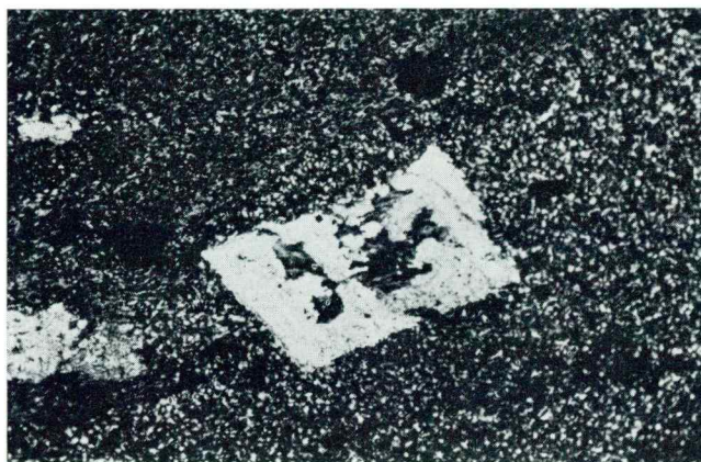
Sl. 8. Idiomorfni siderit (sredina slike) z vključki kaolinita v mikrokristalnem kaolinitu. Rudno telo Brus, II. obzorje, 2. etaža. Presevna polarizirana svetloba, navzkrižni nikoli, povečava 75 ×
