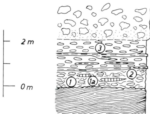
Sl. 24. Litološki presek kaolinitnih usedlin na 7. etaži rudnega telesa Hangend, nad VII. obzorjem
