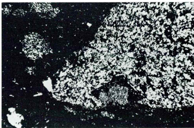
Sl. 19. Isto kot sl. 18, pri navzkrižnih nikolih. Kaolinizirani vtrošnik glincev sestoji iz krypto- in mikrokristalnega kaolinita
