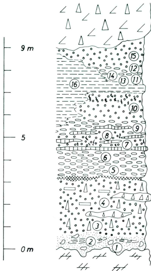
Sl. 25. Litološki presek kaolinitnih usedlin pri slepem jašku št. 16 na II. obzorju Abb. 25. Lithologisches Profil der Tongesteine beim Blindschacht No. 16, II. Sohle 1 pelitska kaolinitna usedlina, 2, 3, 4, 7, 8, 10, 12 in 15 psamitska kaolinitna usedlina, 5, 6, 9, 11, 13 in 14 pšenasta kaolinitna usedlina, 16 peščeni meljevec 1 Tonstein mit pelitischer Struktur, 2, 3, 4, 7, 8, 10, 12 und 15 Tonstein mit psammitischer Struktur, 5, 6, 9, 11, 13 und 14 Graupentonstein, 16 sandiger Siltstein
