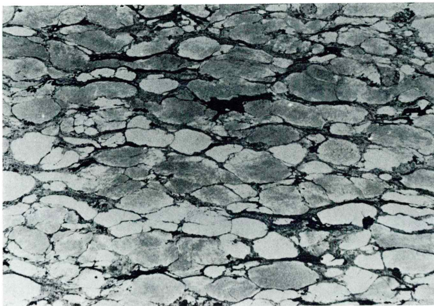
Sl. 4. Debelozrnato kaolinitno usedlino grade predvsem zrna s pšenastim in eliptičnim presekom; veziva je le malo. Črno je pirit. Presevna polarizirana svetloba, povečava 5×. Rudno telo Hangend, VII. horizont, 7. etaža, vzorec 3
