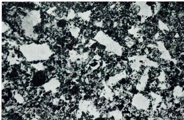
Sl. 22. Kaolinizirana zrna glincev (belo) v kaolinitno-karbonatnem vezivu (sivo). Drobna črna zrnca so pirit. Pri slepem jašku št. 16., II. obzorje, vzorec 4. Presečna polarizirana svetloba, povečava 30 ×
