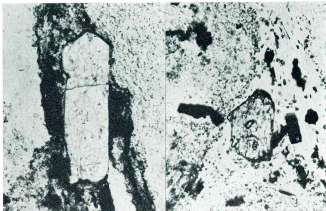
Sl. 15 levo. Kristal apatita v vezivu. Rudno telo Hangend, VII. obzorje, 7. etaža, vzorec 3. 15 desno. Kristal cirkona v vezivu. Pri sipki Bončina, III. obzorje, vzorec 4. Presevna polarizirana svetloba; povečava 200 ×
