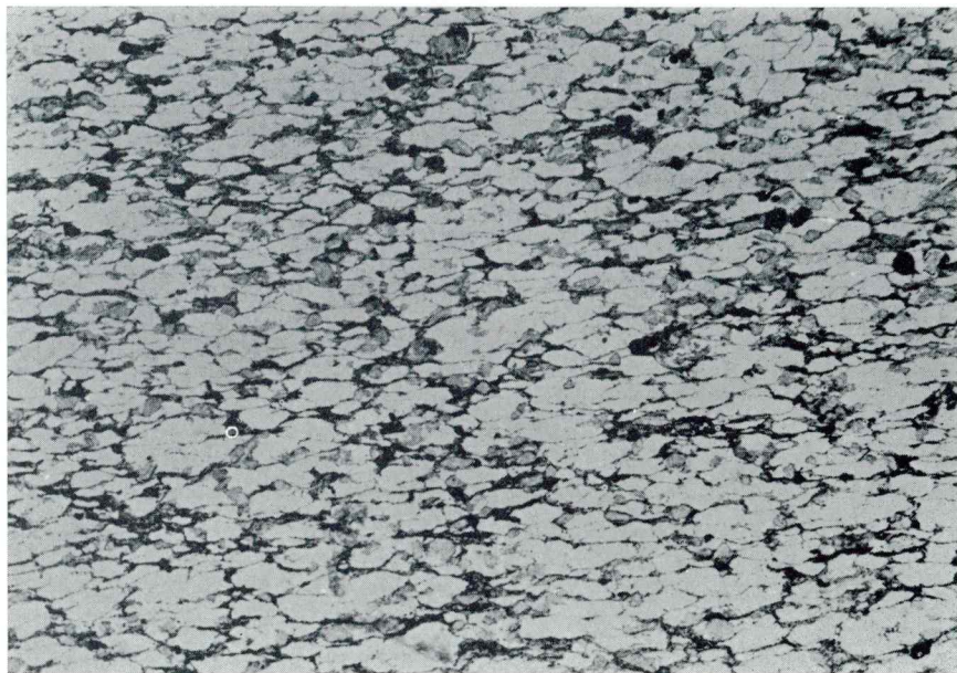
Sl. 5. Srednjezrnata kaolinitna usedlina s pšenasto strukturo. Vezivo je sivo, piritna zrna pa so črna. Pri slepem jašku št. 16, II. obzorje, vzorec 5. Presevna polarizirana svetloba, povečava 7 ×
