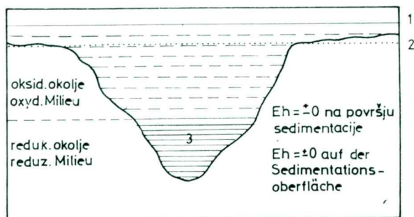
Sl. 19. Redoks \pm 0 nivo glede na površino sedimentacije pri nastanku laminarnega rudonosnega dolomita.
