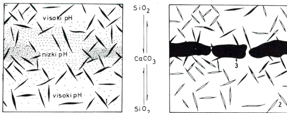
Sl. 11. Nastanek rožencev iz kremenastih spikul po Newellu in sod. (1953)
