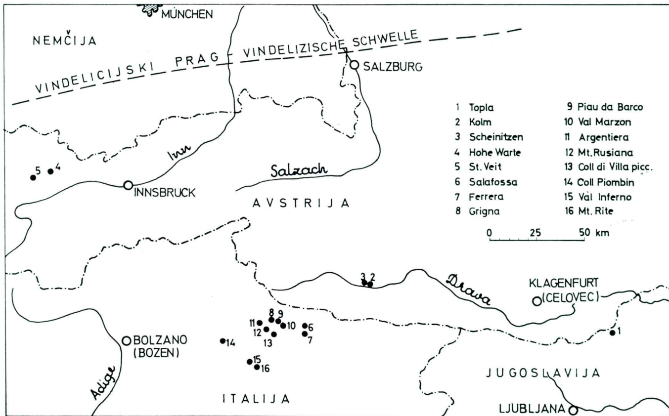
Sl. 21. Anizična svinčevo-cinkova rudišča na območju Vzhodnih Alp
