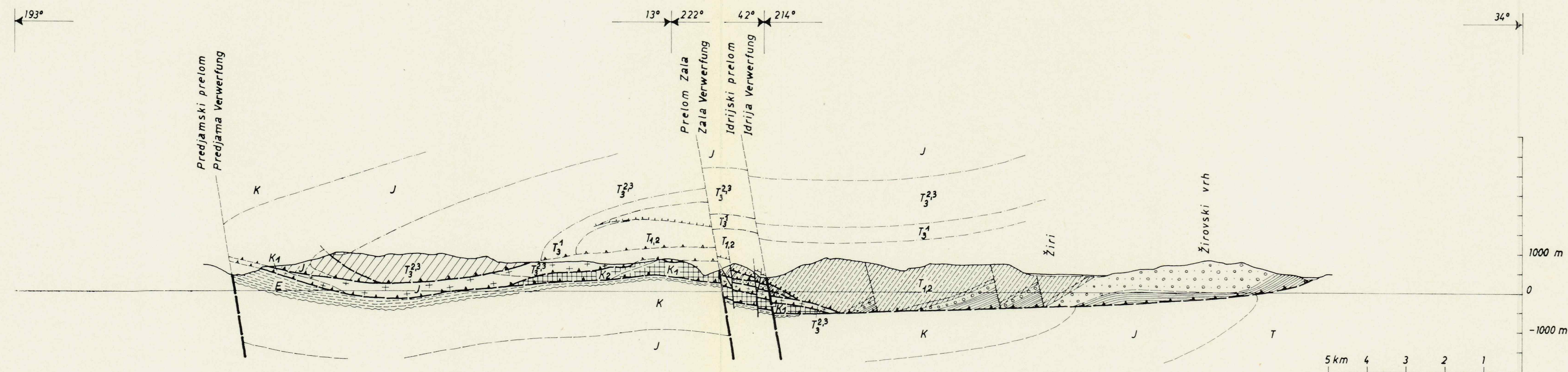
Sl. 2 Sedanja lega krovnih enot. Dopolnjen MLAKARJEV profil (1969, 2.sl., profil C) – Abb. 2 Gegenwärtige Lage der Deckeneinheiten. Ergänzttes Profil von MLAKAR (1969, 2.Abb., Profil C)
