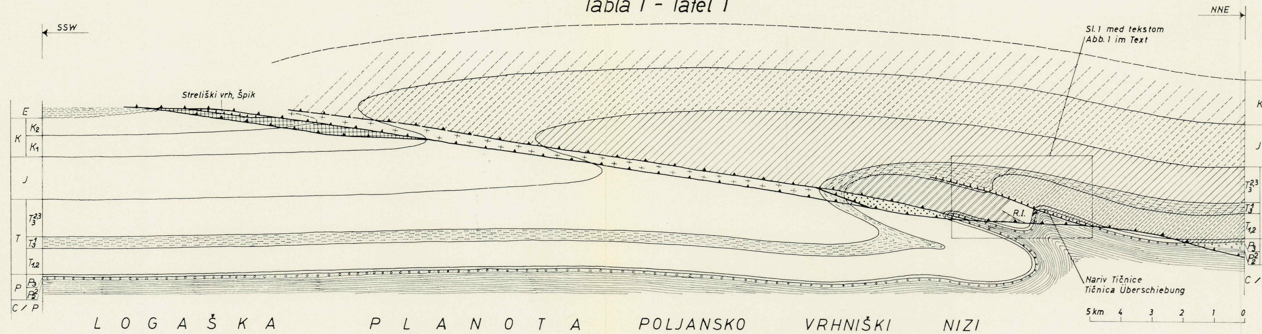
Sl. 1 Izhodna struktura polegla gube s prvotno lego krovnih enot – Abb. 1 Die Ausgangsstruktur der liegenden Falte mit ursprünglicher Lage der Deckeneinheiten
