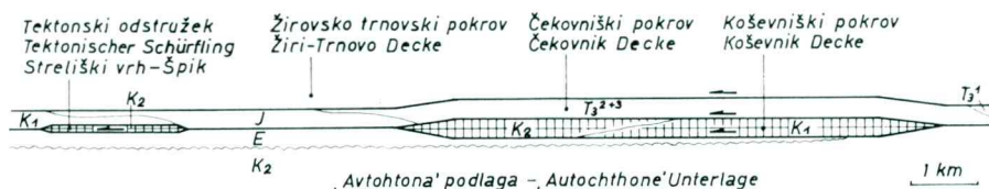
Sl. 3. Lega Špika in Streliškega vrha v krovni zgradbi idrijsko žirovskega ozemlja Abb. 3. Die Lage von Špik und Streliški vrh im Idrija-Žiri Deckenbau
