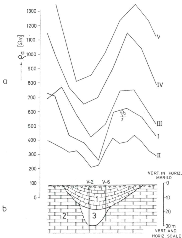
Sl. 2. Rezultati poizkusnih geoelektričnih raziskav na krpi eocenskega apnenca a Diagrami navidezne specifične upornosti Q_a , I Schlumbergerjeva razvrstitev AB = 70 m, MN = 10 m, II Wennerjeva razvrstitev a = 10 m, III Wennerjeva razvrstitev a = 20 m, IV Wennerjeva razvrstitev a = 30 m, V Wennerjeva razvrstitev a = 40 m
