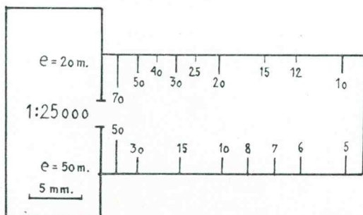
Sl. 6. Enostaven merilnik razdalj.
