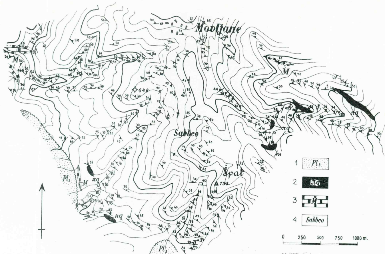
Sl. 9. Detajl klasične geološke karte (list ORAHOVAC 54); na njem je paleozojska formacija prikazana samo z znaki za vpad foliacije. 1. zgornjepliocenski sedimenti, 2. kremenov porfir, 3. marmor, 4. albitno-biotitno-kloritni skrilavec.
