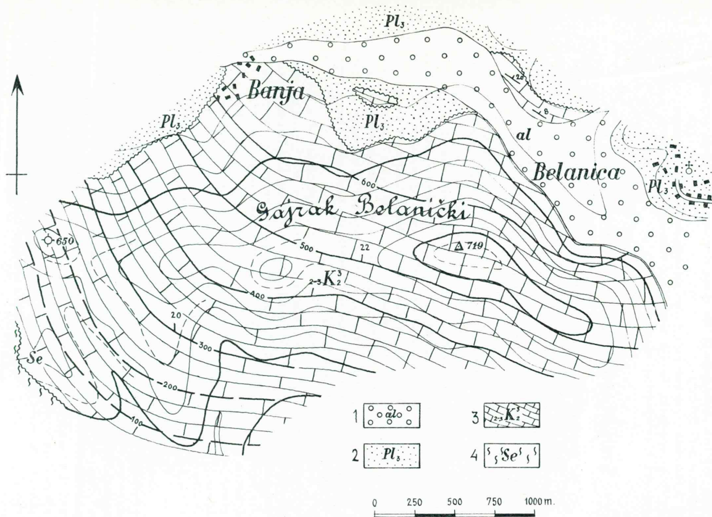
Sl. 12. Detajl geološke karte lista ORAHOVAC 54.1; tektonska struktura in debelina senonskega plastovitega apnenca sta prikazani z izostratami.
