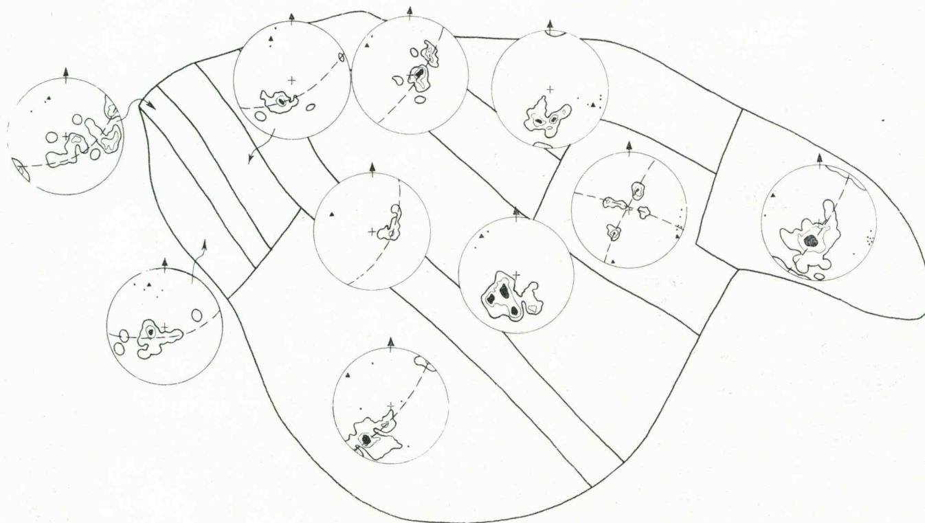
Sl. 10. Isto območje kot na sl. 9. Konturni diagrami foliacije za homogena polja s poli statistične osi B in lineacije.
