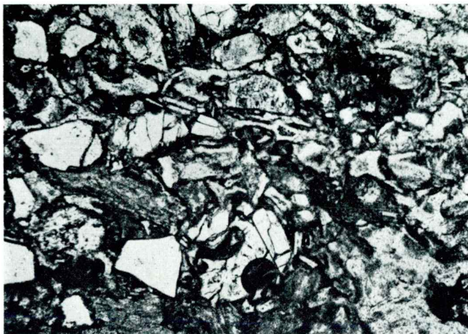
Sl. 9. Vz. 4 567/11 586, jugozahodno od Št. Ruperta. Nikola //, 35 X. Andezitni kristalo- in litoklastični tuf z značilnimi steklastimi kameninskimi fragmenti
