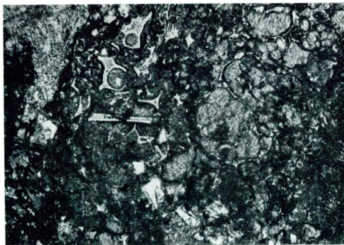
Sl. 10. Vrtina 1/61, Mala Pirešica, vz. 1/7 249, gl. 101,20 m, nikola //, 35 X. Lapilni andezitni tuf s fragmenti plovca in značilnimi drobci stekla
