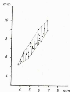
Sl. 7 b. Amphimelania holandri (Férussac); na abscisi ŠU, na ordinati VU
