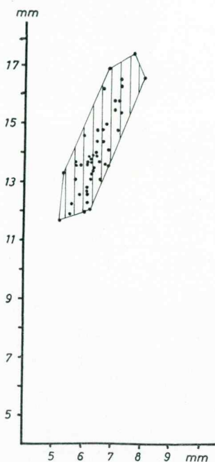
Sl. 6 a. Fagotia esperi (Férussac); na abscisi ŠH, na ordinati VH
