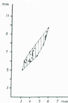
Sl. 1 b. Lymnaea peregra lagotis (Schränk); na abscisi SU = širina ustja; na ordinati VU = višina ustja
