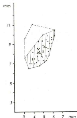
Sl. 5 b. Fagotia acicularis (Férussac); na abscisi ŠU, na ordinati VU
