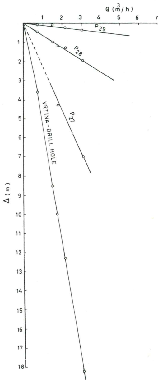
Sl. 5. Diagram odvisnosti depresije \Delta od količine črpane vode Q v vrtini in piezometriških cevah
