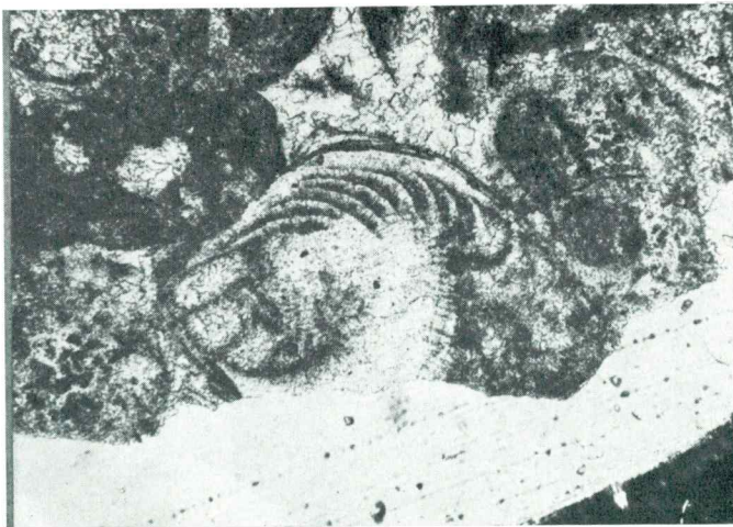
Sl. 4b. Protopeneroplis striata Weynschenk, 75 \times , spodnji malm, Zagradec-Randol št. zb. 23—12434
