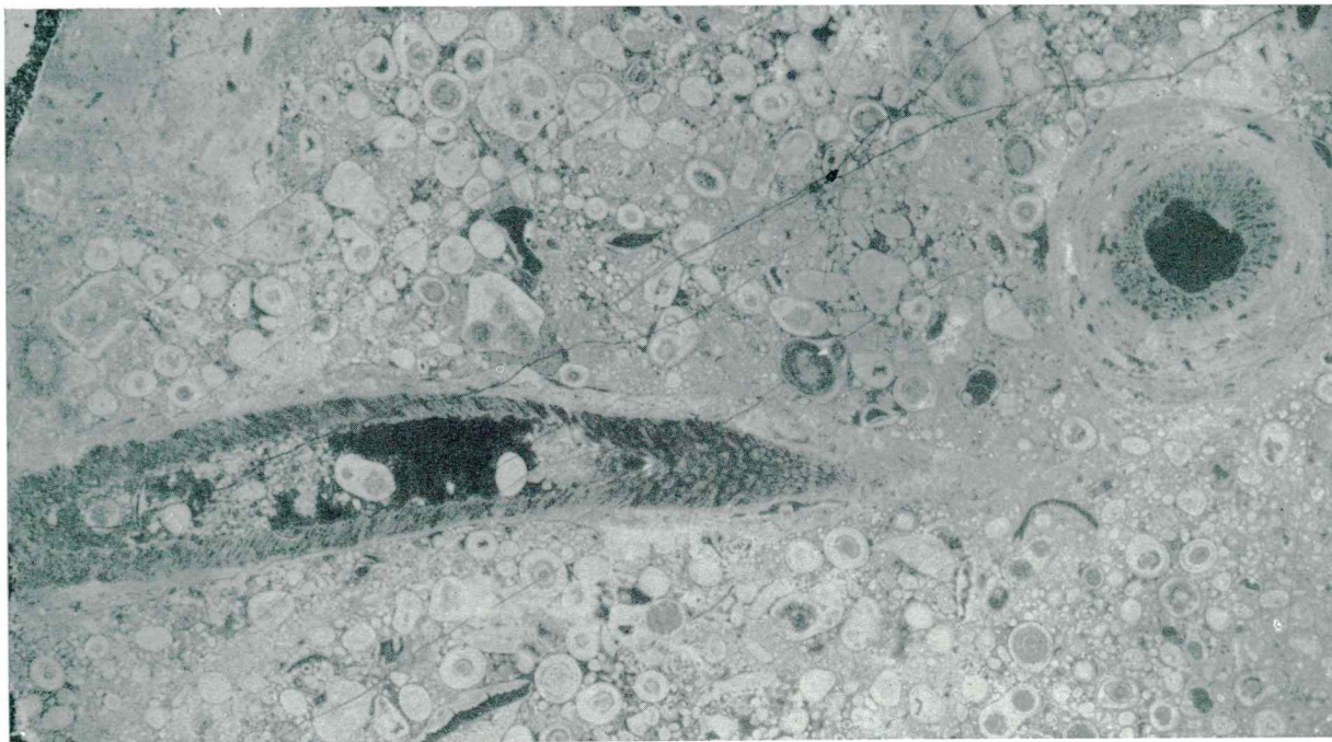
Sl. 1. Palaeodasycladus mediterraneus (Pia), 8×, spodnja liada, Zagradec—Randol, št. zb. 1144—6912
