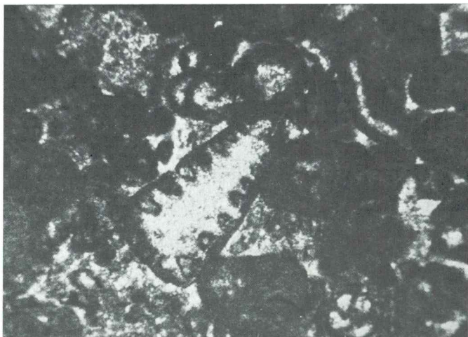
Sl. 5. Coscinococonus sp., 35 X, spodnji malm, Zagradec-Randol, št. zb. 711—6761
