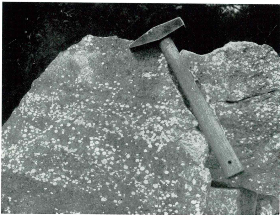
2. sl. Keramosferine v apnencu iz okolice Dutovelj
