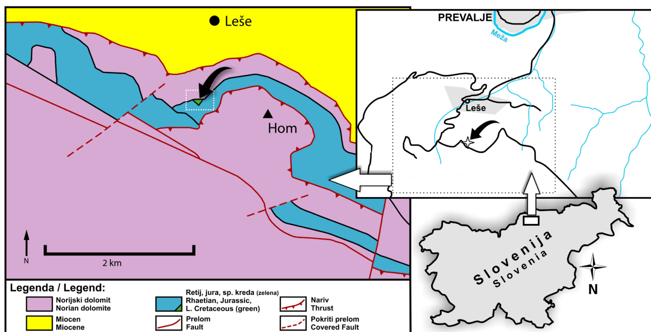
Sl. 1. Geografska lega in poenostavljena geološka karta okolice najdišča spodnjekredne favne pri Lešah. Prirejeno po Ramovš & Rebek (1970).
