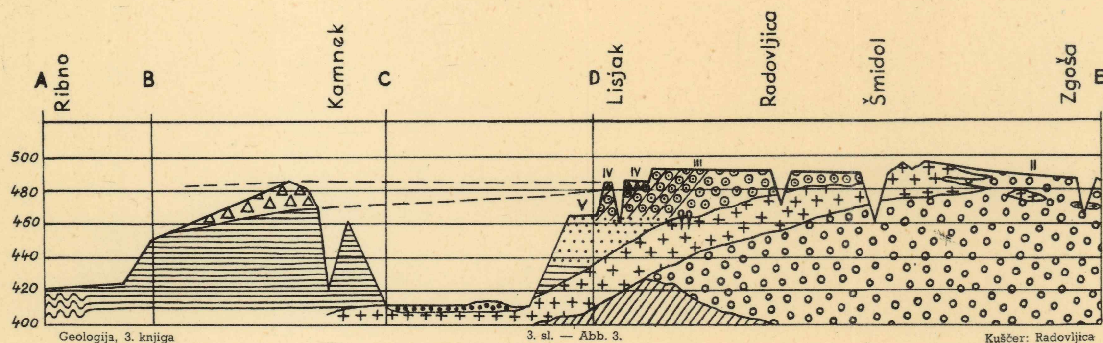
Profil Ribno — Zgoša v južnem delu radovljiške kotline (A—B—C—D—E na 1. sl.) Profil von Ribno bis zur Zgoša im südlichen Teil des Beckens von Radovljica (A—B—C—D—E auf Abb. 1.)
