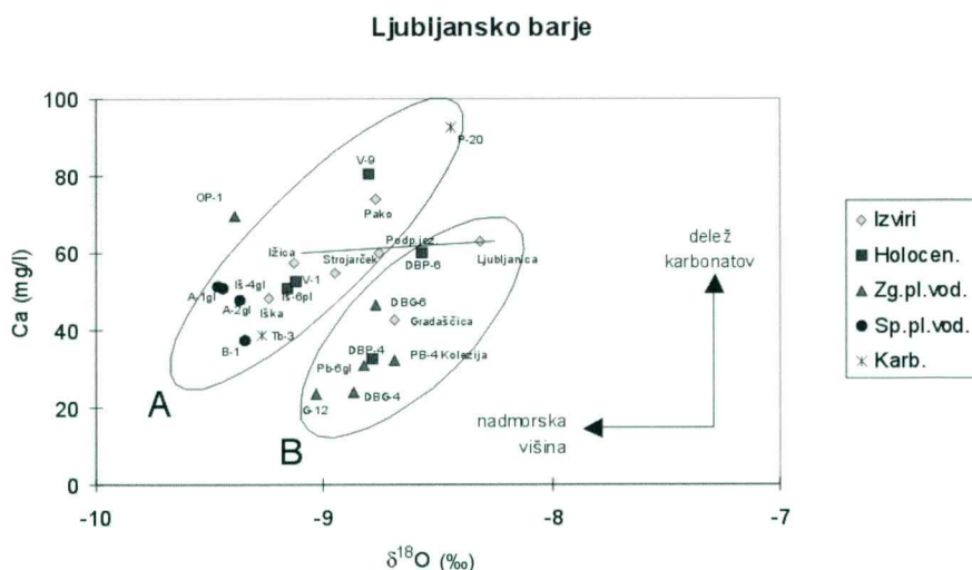
Slika 5: Razmerje med povprečno izotopsko sestavo kisika in povprečno koncentracijo kalcija v podzemnih in površinskih vodah Ljubljanskega barja
