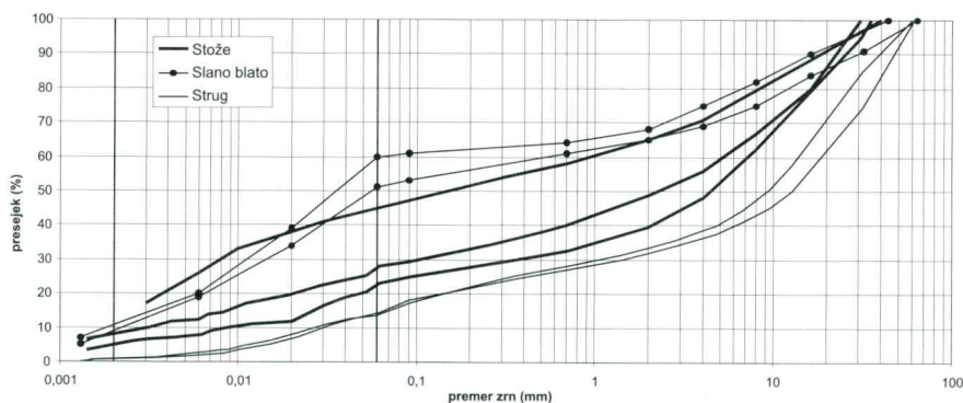
Slika 2: Krivulje zrnavosti za plazine iz plazov Stože, Slano blato in Strug
