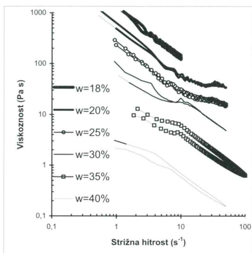
Slika 4: Rezultati viskozimetra: frakcija do 63 mm s plazju Stože
