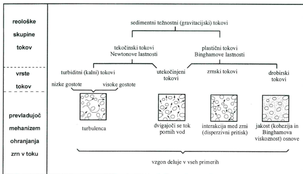
Slika 1: Sedimentno težnostni tokovi in prevladujoči mehanizmi ohranjanja zrn v toku (privzeto iz Škaberne, 2001).
