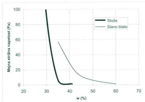
Slika 8: V viskozimetru določena mejna strižna trdnost v odvisnosti od vlažnosti za materiala s plazov Stože in Slano blato
