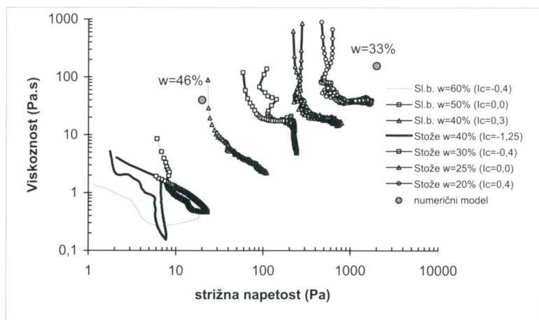
Slika 6: V viskozimetru ugotovljen odnos med viskoznostjo in strižno napetostjo za materiala s plazju Stože in Slano blato ter podatka, dobljena s povratno numerično analizo drobirskih tokov 15. in 17. 11. 2002 izpod Stožja.
