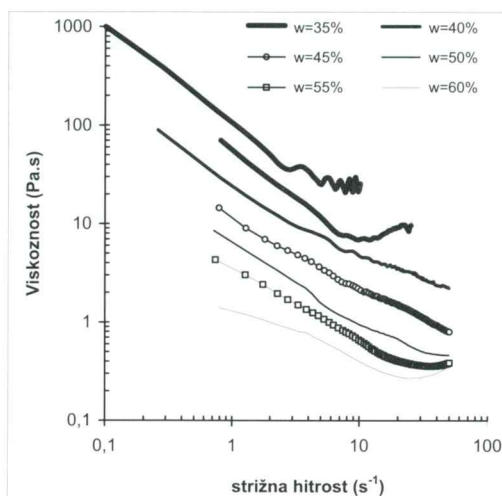
Slika 5: Rezultati viskozimetra: frakcija do 63 mm s plazju Slano blato
