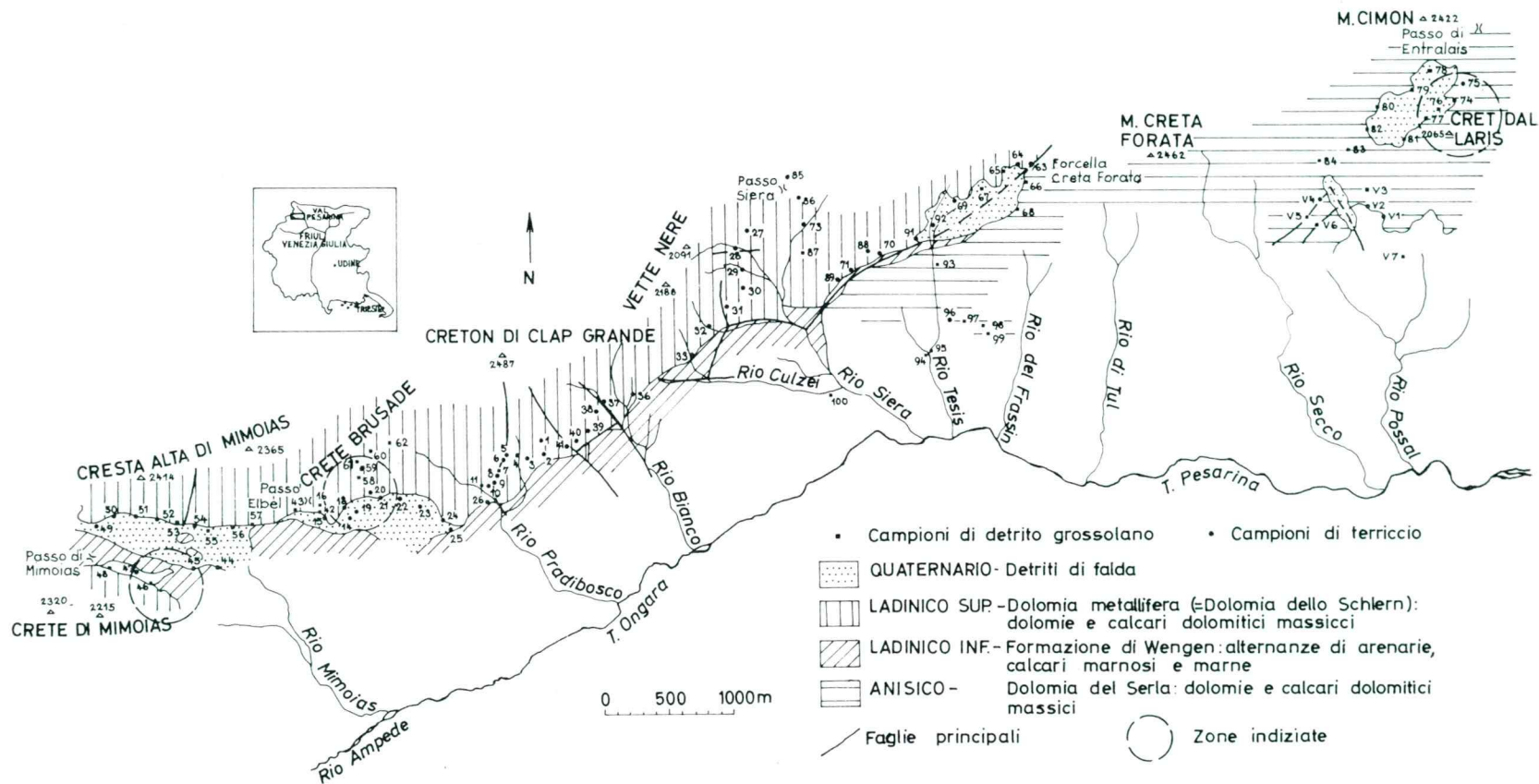
Fig. 2. Schema geologico preliminare del versante sinistro dell'alta e media Val Pesarina con l'ubicazione dei campioni geochimici
