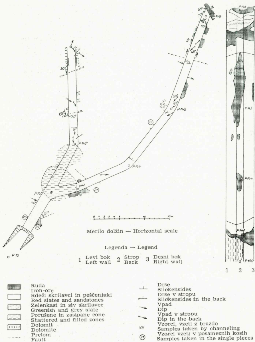
2. sl. Jamska karta rova Močile Fig. 2. Mine map of the Močile adit
