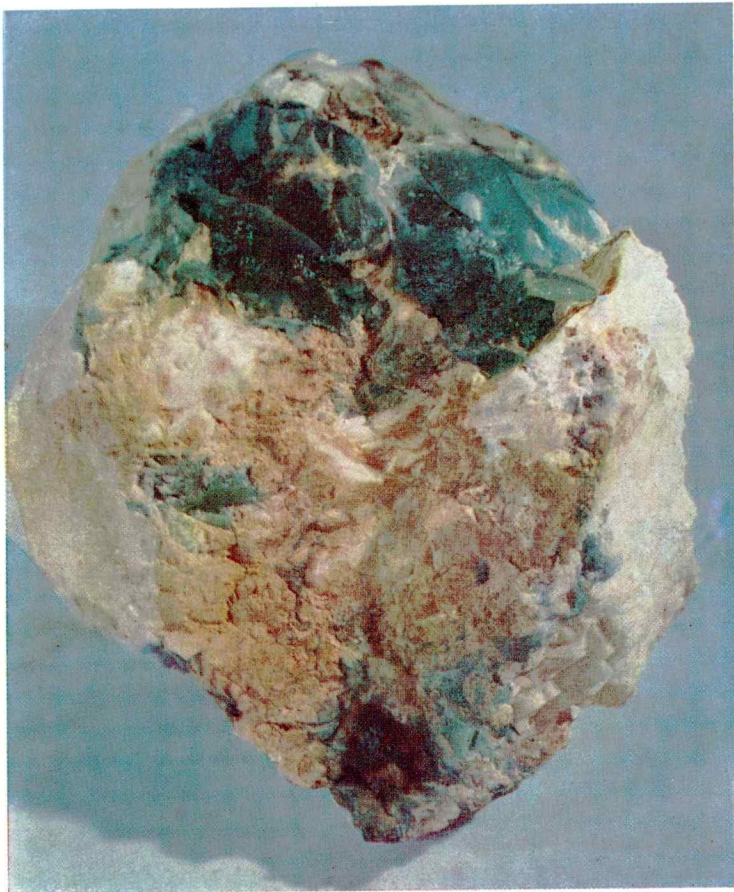
PARAGONIT V DOLOMITNEM MARMORJU IZ KRAJA CVETKOVO GJUBRIŠTE, MAKEDONIJA \frac{1}{2} NARAVNE VELIKOSTI
