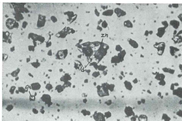
3. sl. Mežica—Topla. Zraščenje sfalerita (zn) z dolomitom (d) v flotacijskem materialu. Ultropak, 200 × povečano.
