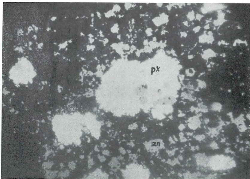
2. sl. Mežica—Topla. Drobnno zrnat sfalerit (zn) zrasel s piritom (px) in jalo- vino (j). Odb. svetloba, oljna imerzija, 50 × povečano.
