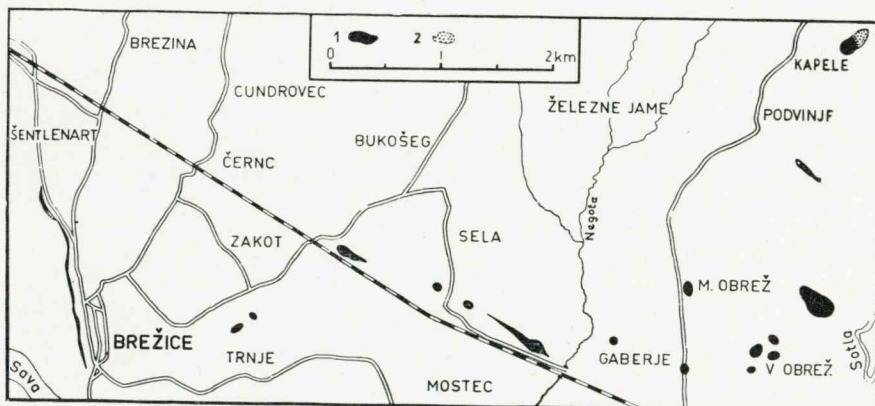
1. sl. Skica srednjepanonskih plasti med Šentlenartom in Velikim Obrežem. 1 glineni in peščeni laporji, 2 drobno zrnati kremenovi peski
