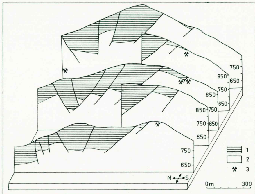
6. sl. Kulisni diagram območja Jankovec—Mučevo
