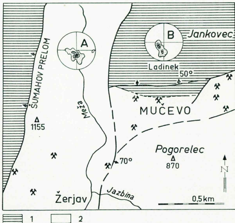
5. sl. Geološka skica raziskovalnega območja Jankovec—Mučevo Bild 5. Geologische Skizze des Untersuchungsgebietes Jankovec—Mučevo
