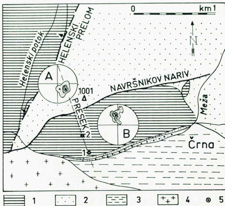
2. sl. Geološka skica raziskovalnega območja Pristava pri Črni Bild 2. Geologische Skizze des Untersuchungsgebietes Pristava bei Črna
